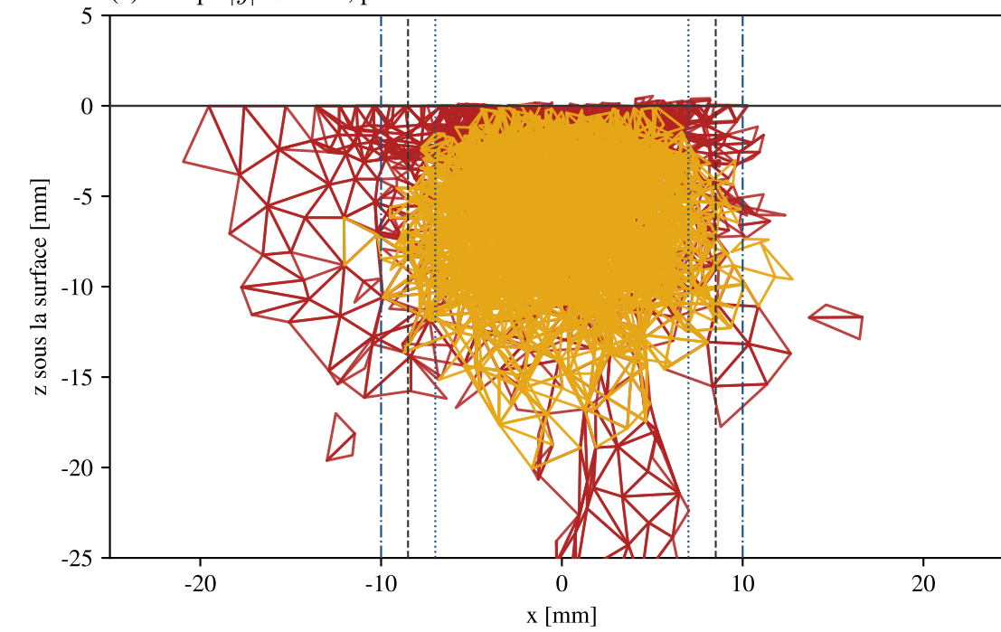
(c) Coupe |y| < 5 mm, par mode
