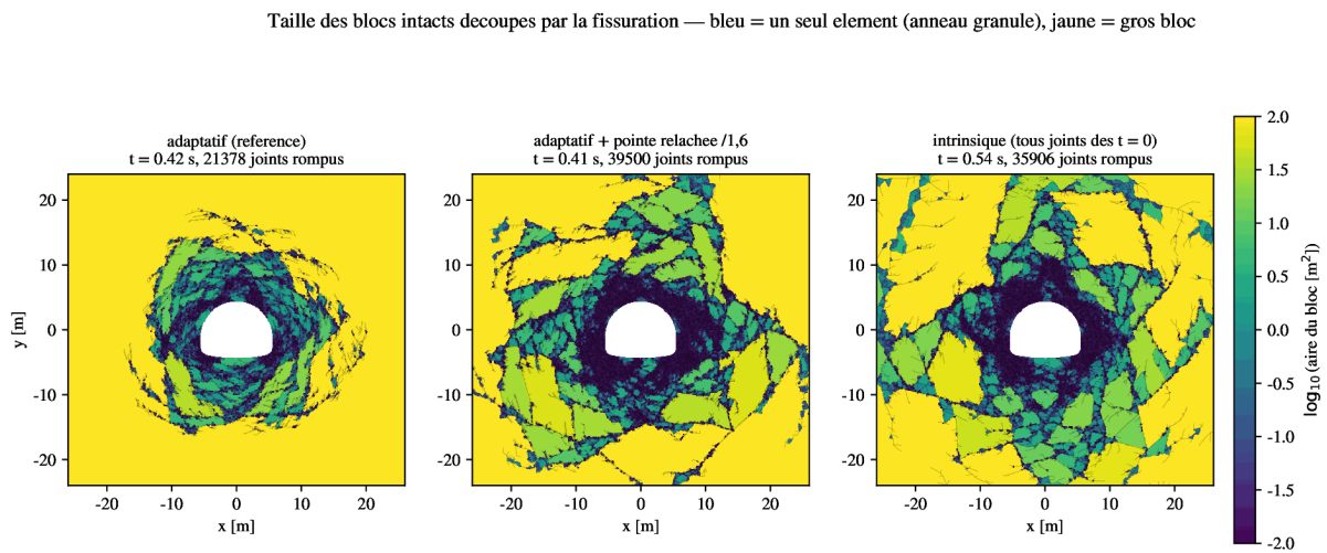
FIGURE 39 – Taille des blocs intacts (aire en échelle logarithmique) pour l'insertion adaptative, l'adaptative avec k_{\text{tip}} = 1,6 et l'intrinsèque : l'adaptative granule un anneau, les deux autres découpent des blocs polygonaux de quelques dizaines à quelques centaines de m 2 .
