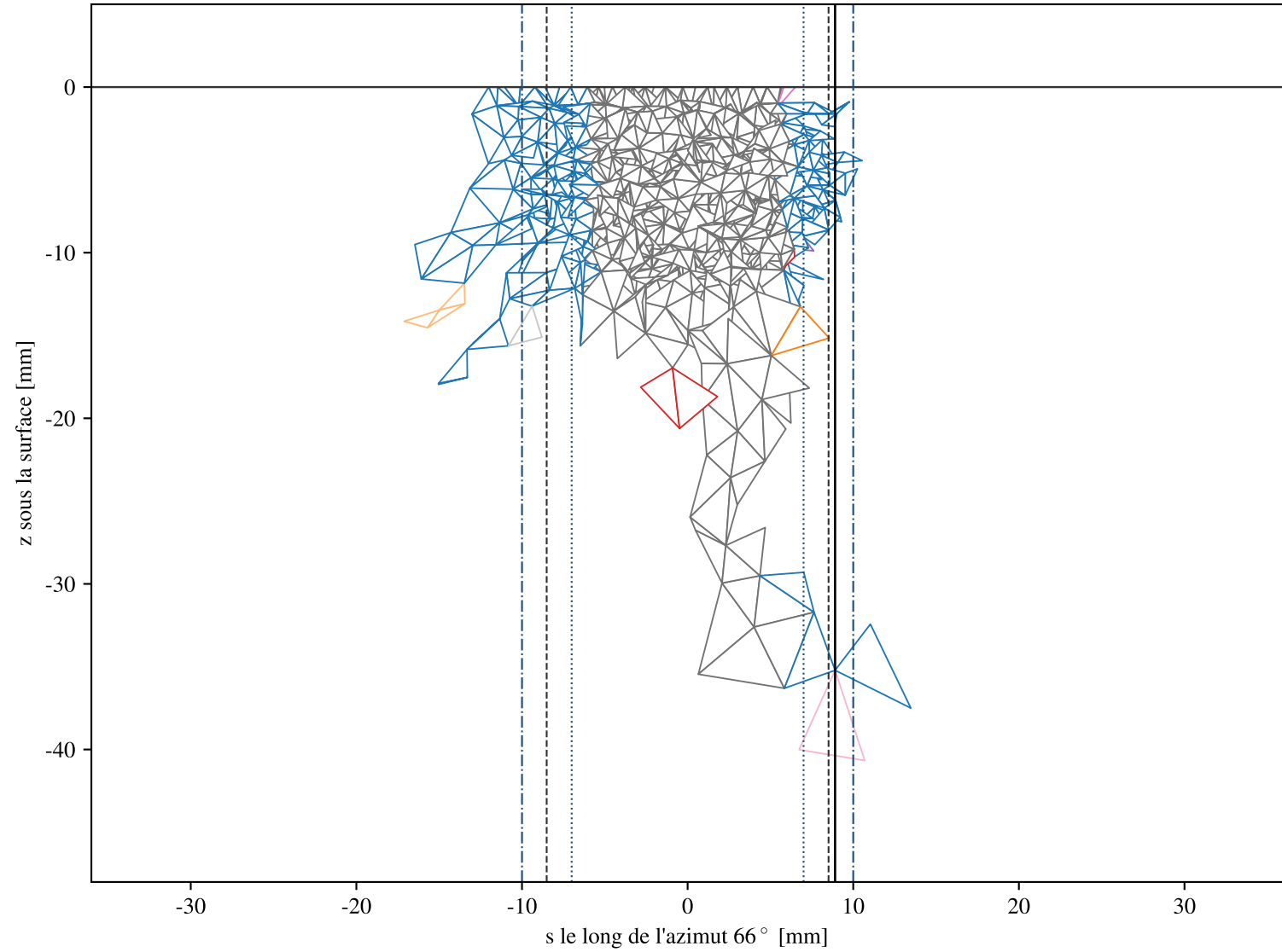
(b) coupe verticale par l'axe et la pointe radiale, |d| < 1.5 mm
