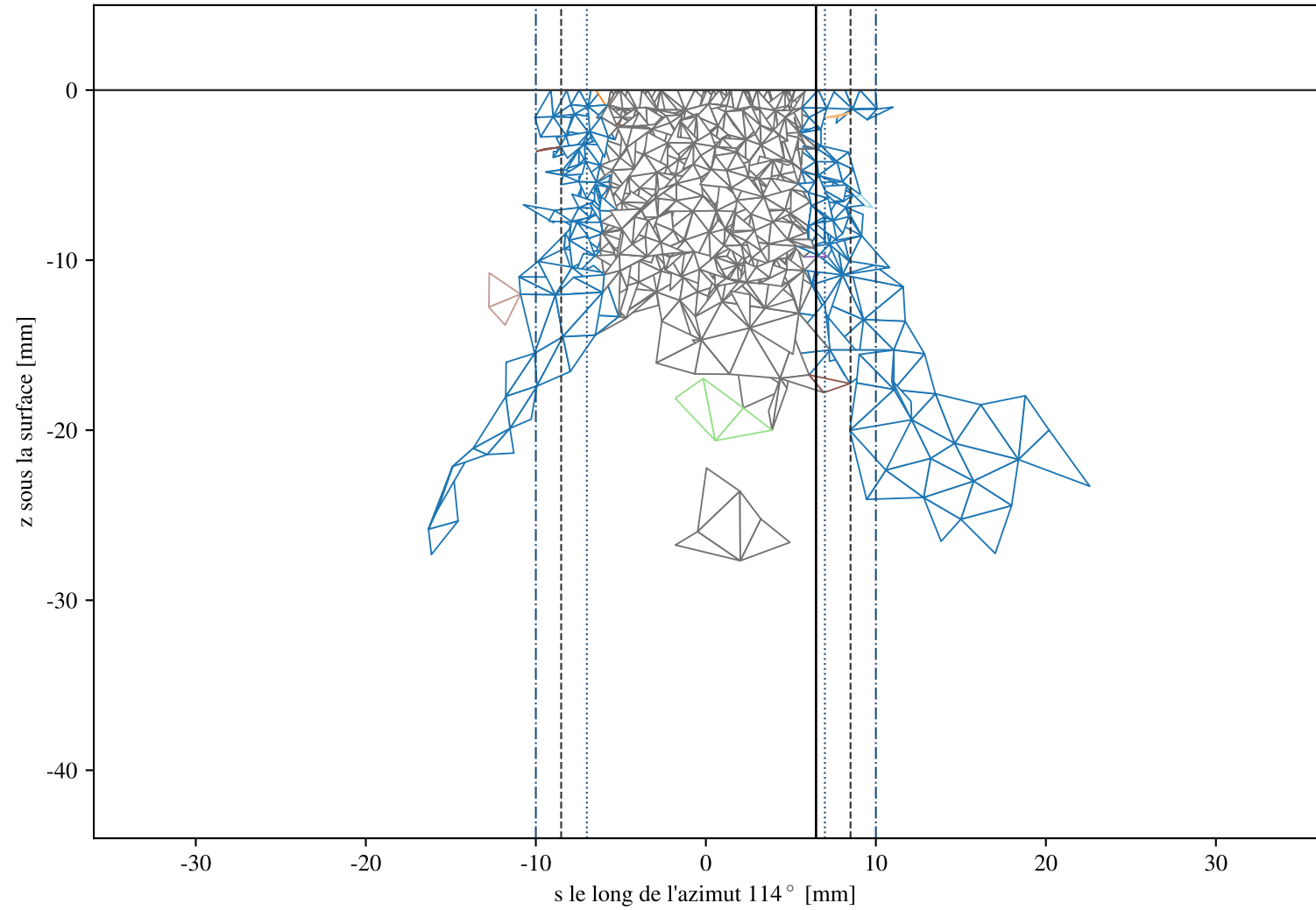
(b) coupe verticale par l'axe et la pointe radiale, |d| < 1.5 \text{ mm}
