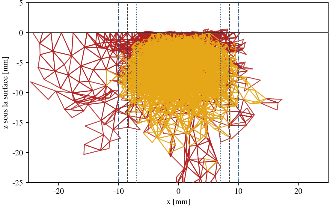
(c) Coupe |y| < 5 mm, par mode
