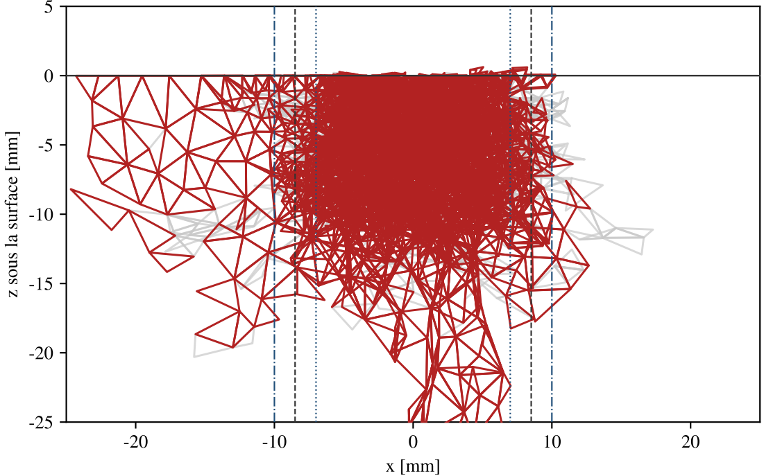
(f) Coupe |y| < 5 mm — fissures / broye
