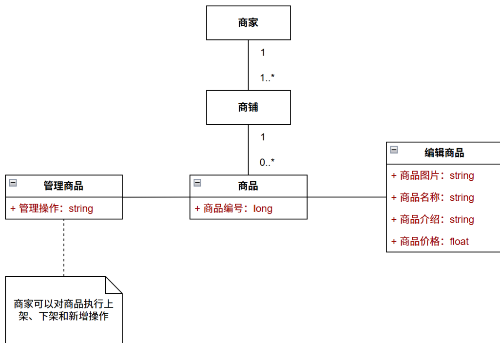
图 1-3 商品管理类图
