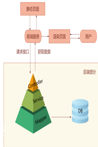
图 1-15 系统技术架构
