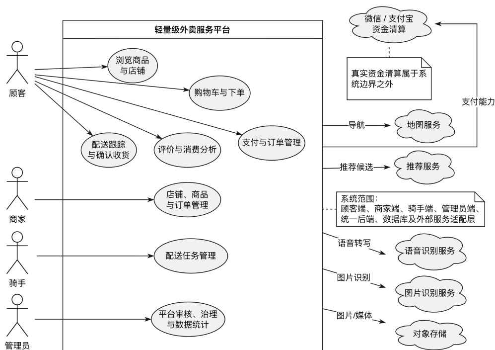
图 1-1 系统上下文图
