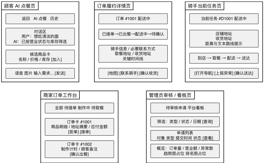
图 1-17 关键页面低保真原型组
