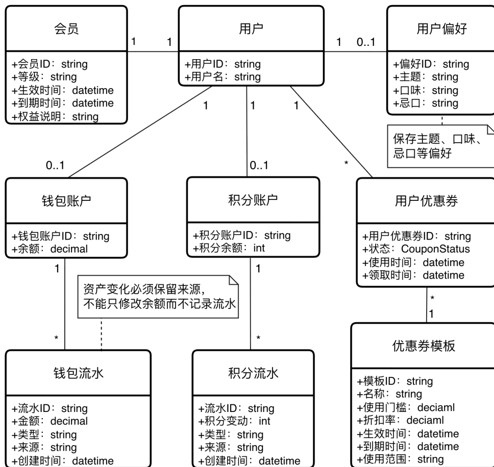
图 1-3 营销资产与智能交互业务概念类图
