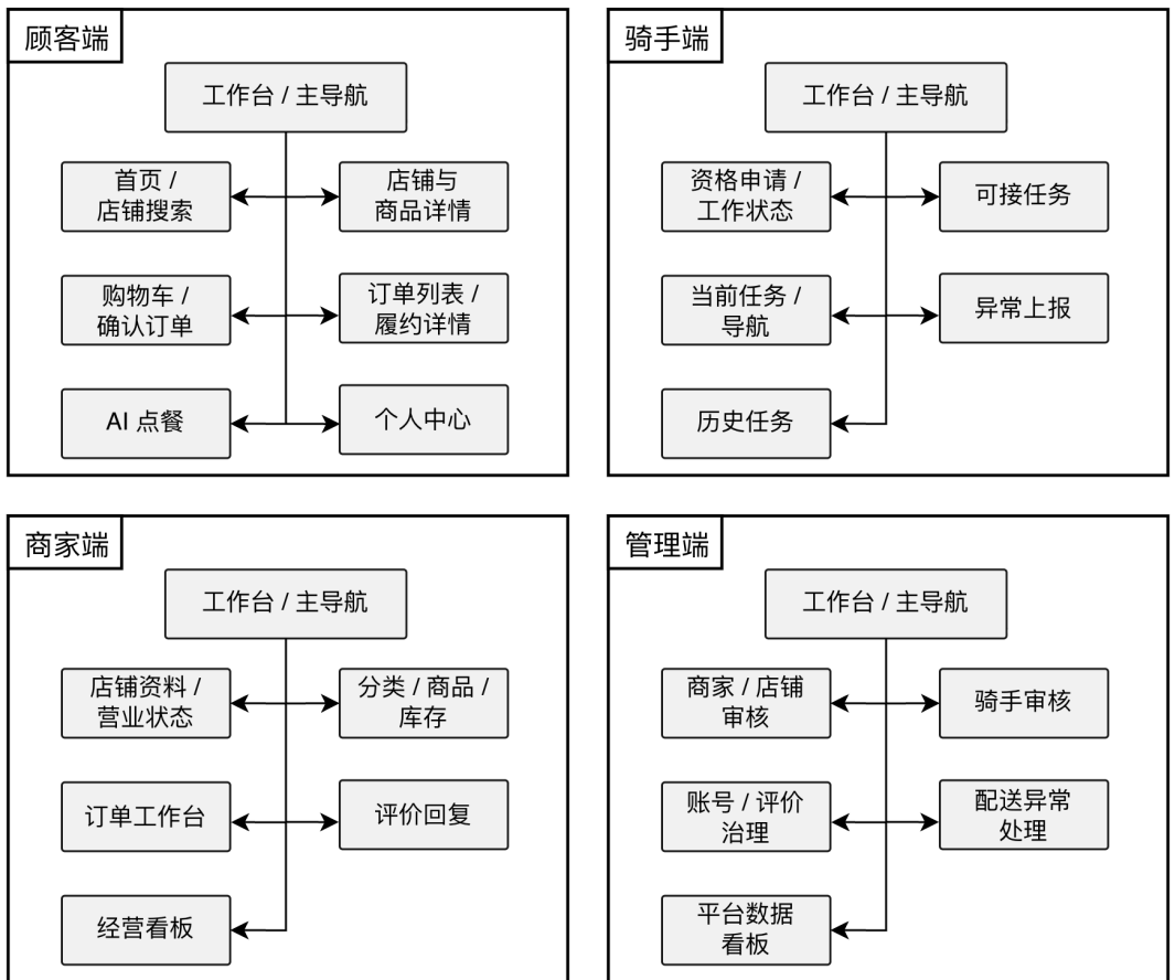
图 1-16 四端页面信息架构图
