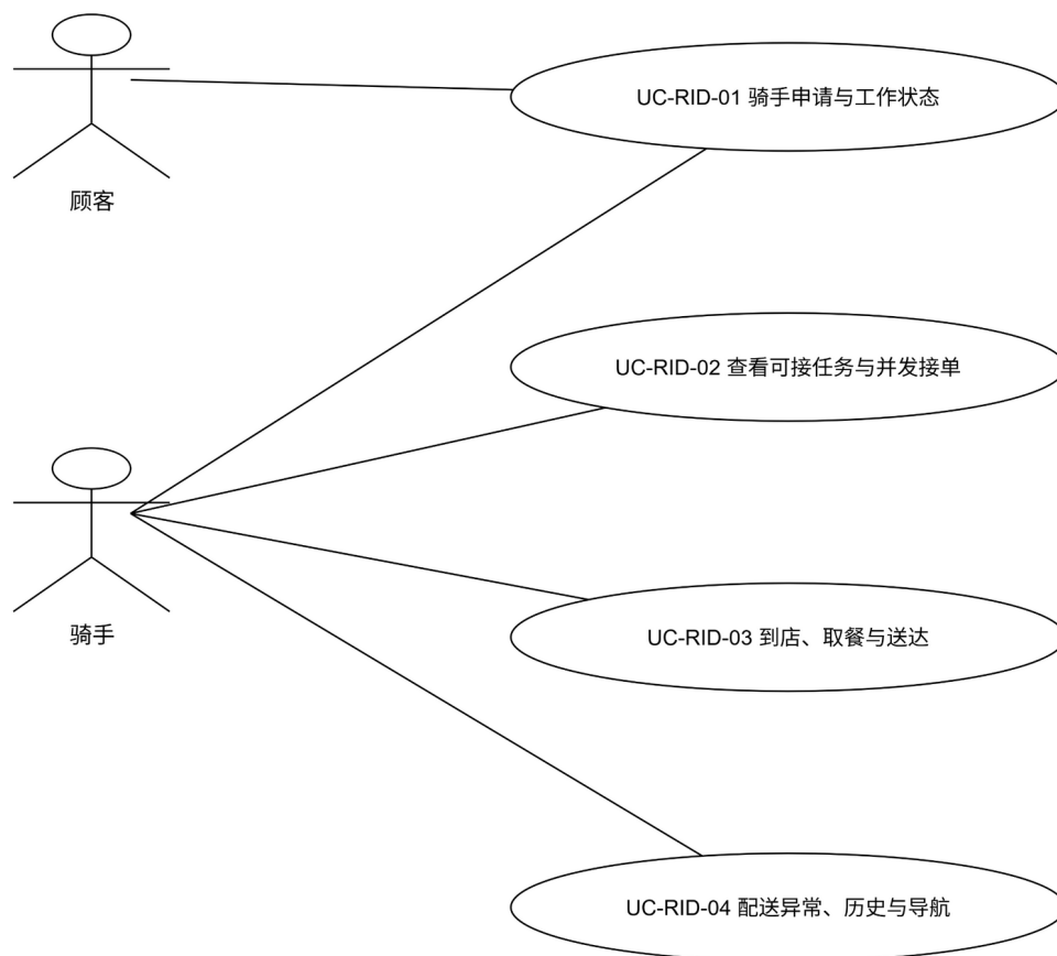
图 1-13 骑手用例图
