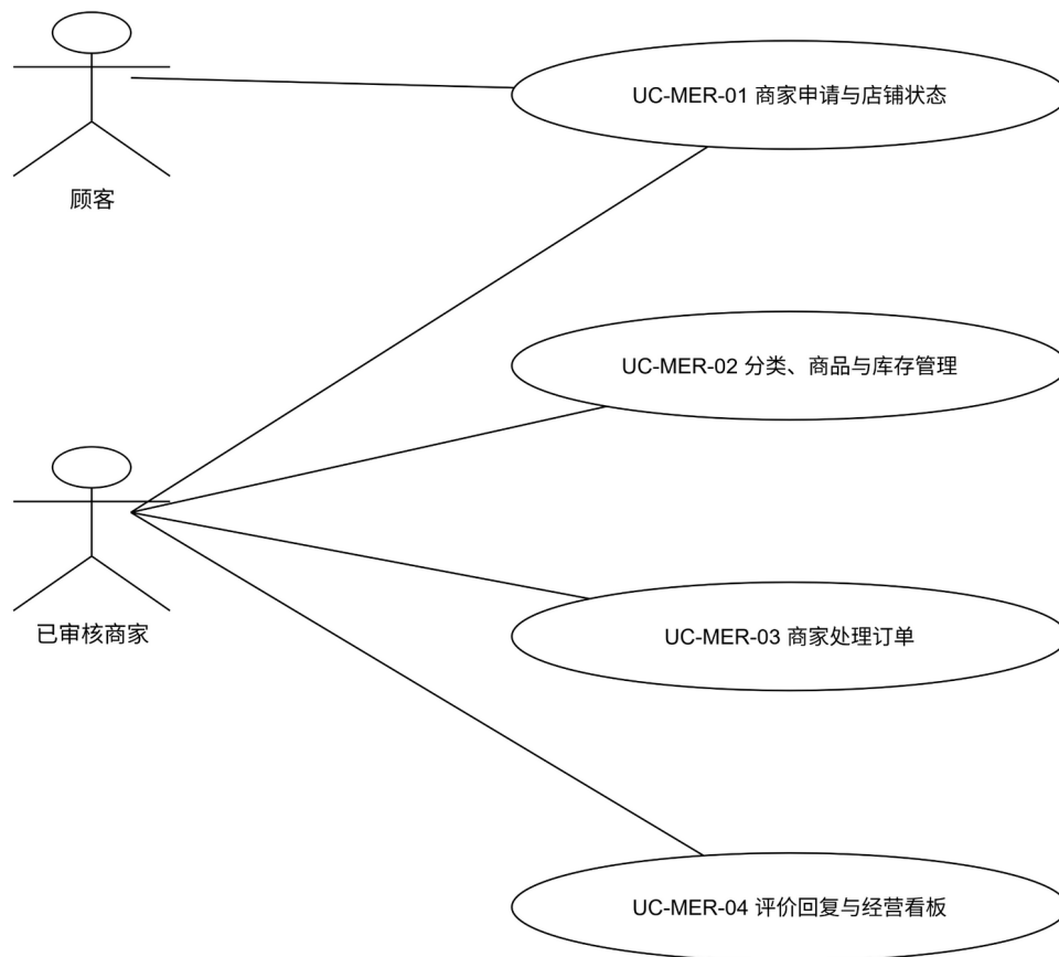
图 1-12 商家用例图
