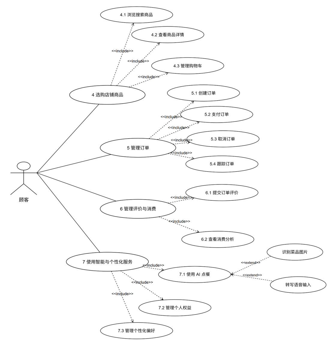
图 1-11 顾客用例图
