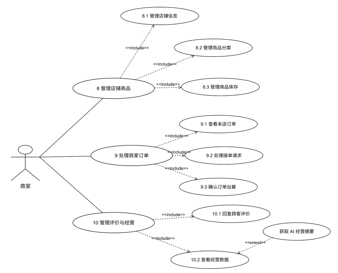
图 1-12 商家用例图
