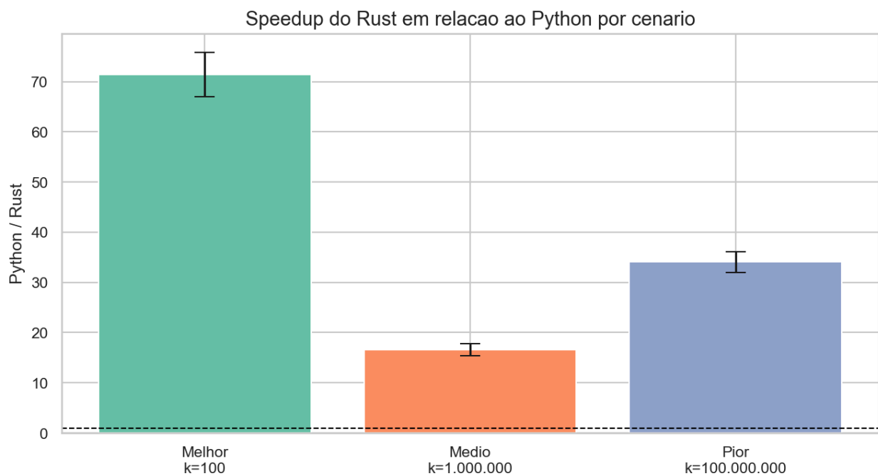
Figura 5 - Speedup do Rust em relacao ao Python por cenario.
