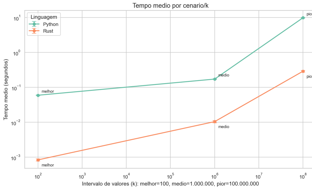
Figura 2 - Tempo medio de execucao por cenario e linguagem.
