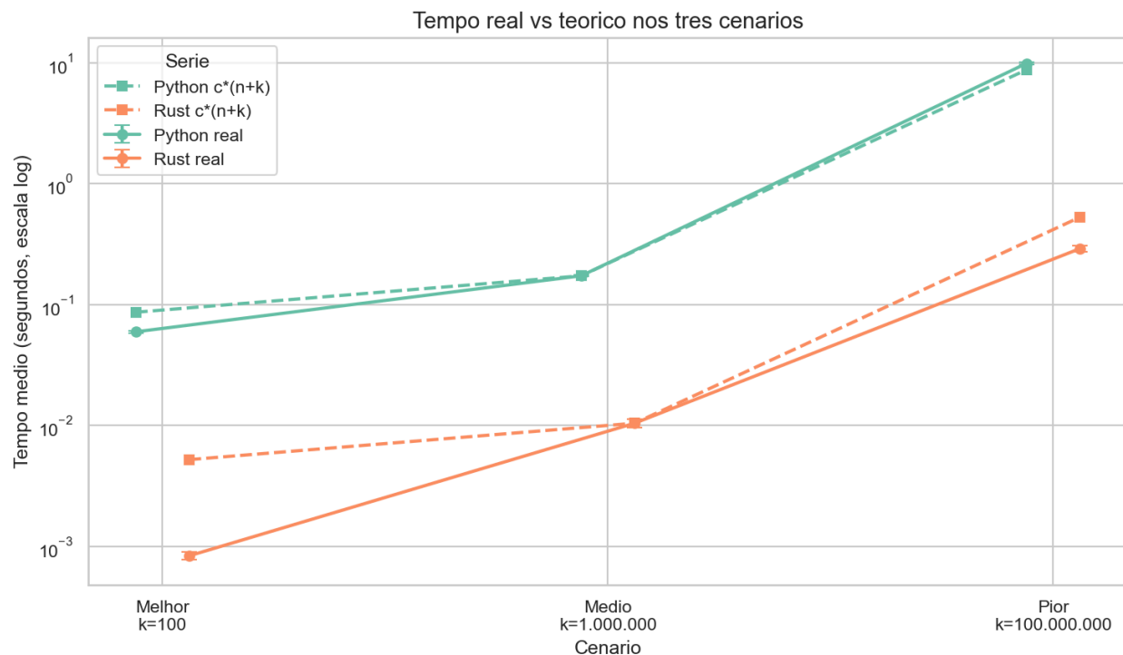
Figura 4 - Comparacao entre tempo real e teorico nos tres cenarios.
