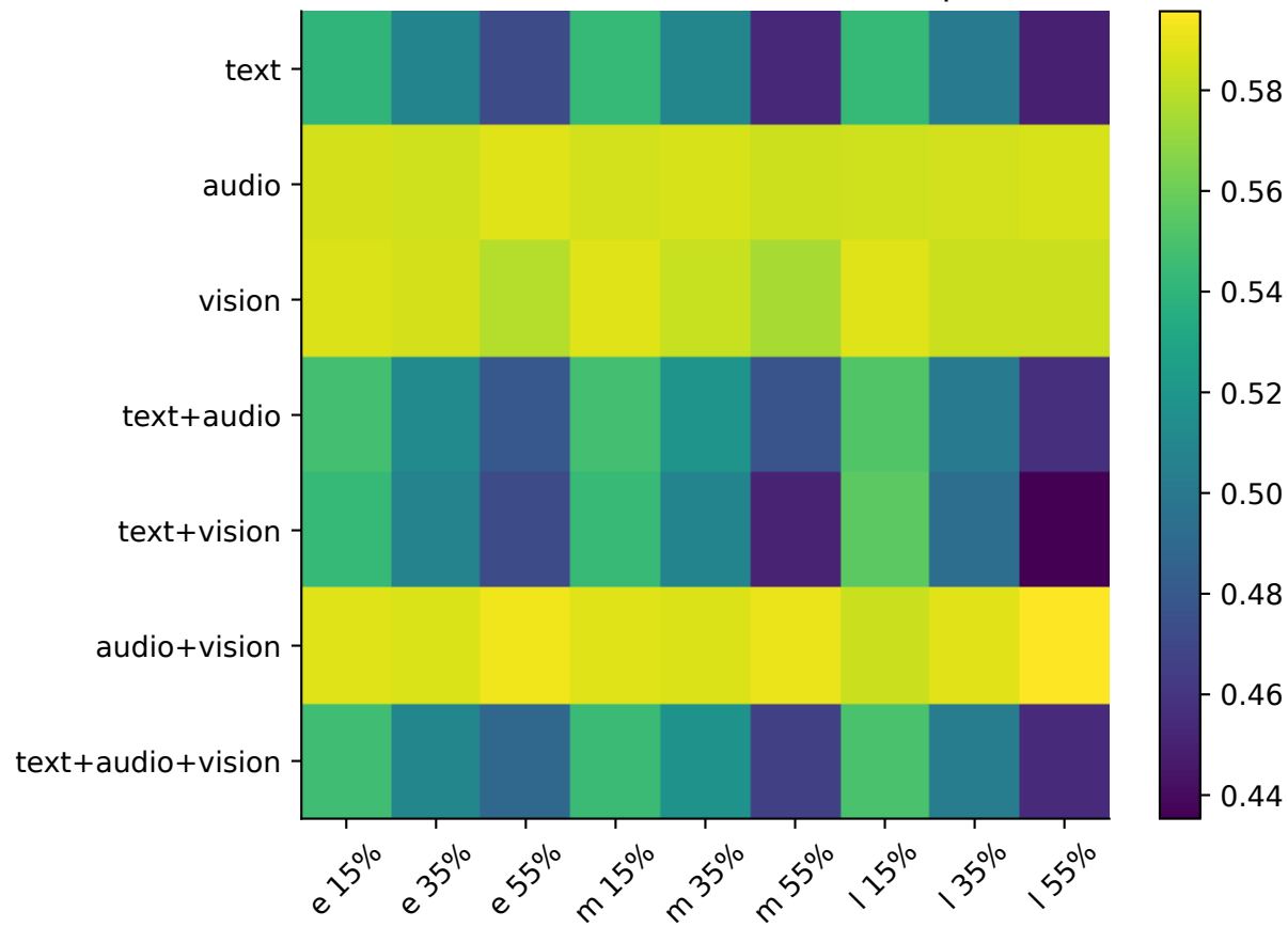
Macro F1 (common feasible samples)
