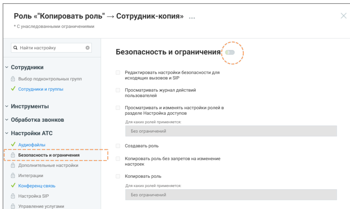
Рисунок 5. Роль-копия, с унаследованными запретами
