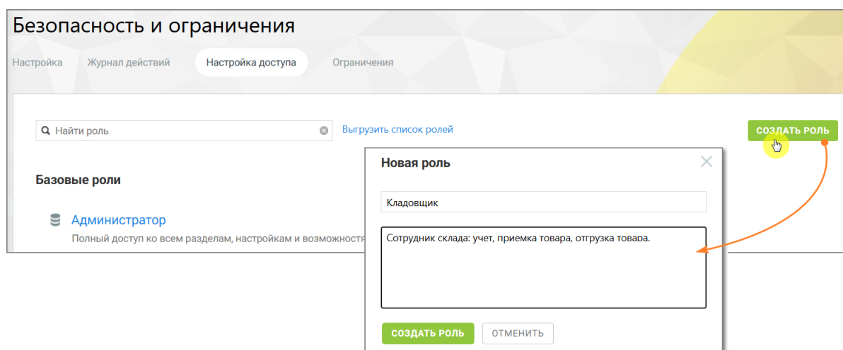
Рисунок 2. Как работает кнопка «Создать роль»
