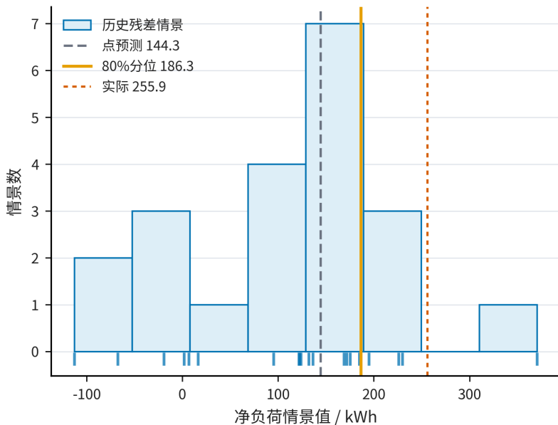
(a) 情景直方图与样本刻度
