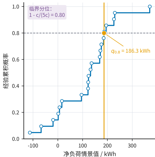
(b) 经验分布函数
