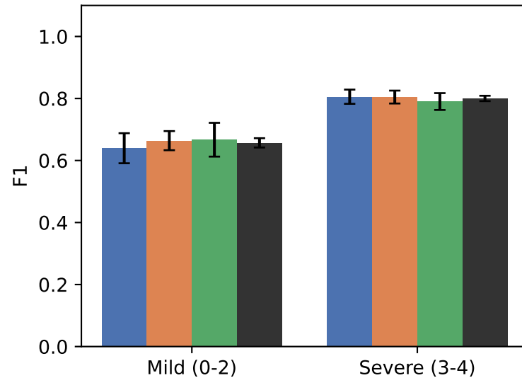
F1
