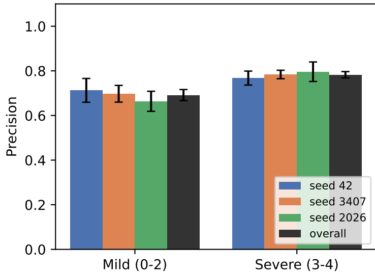
Precision
