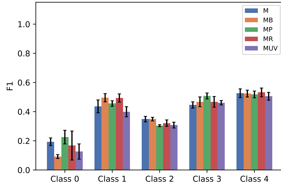
F1
