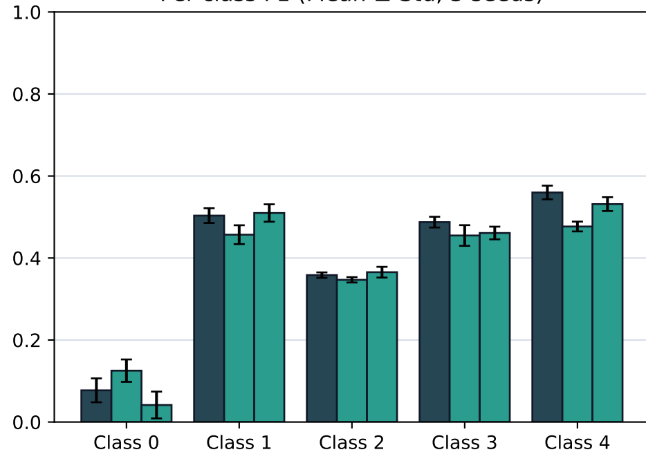
Per-class F1 (Mean \pm Std, 3 seeds)
