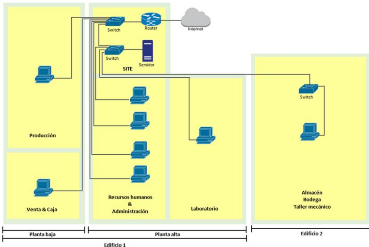
Ilustración 1. Topología física de la red LAN
