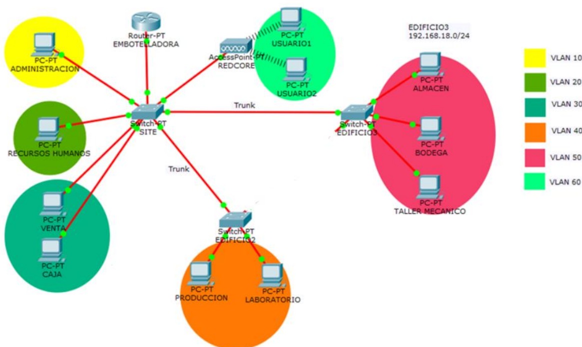
Ilustración 2. Topología física de la sede Guadalajara
