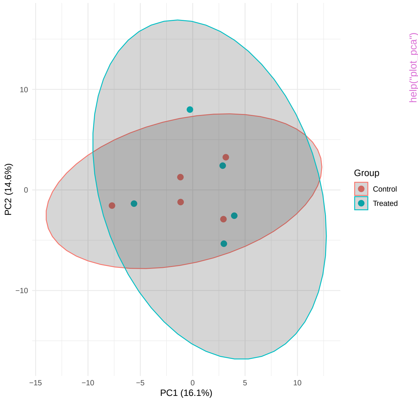
PCA Plot
