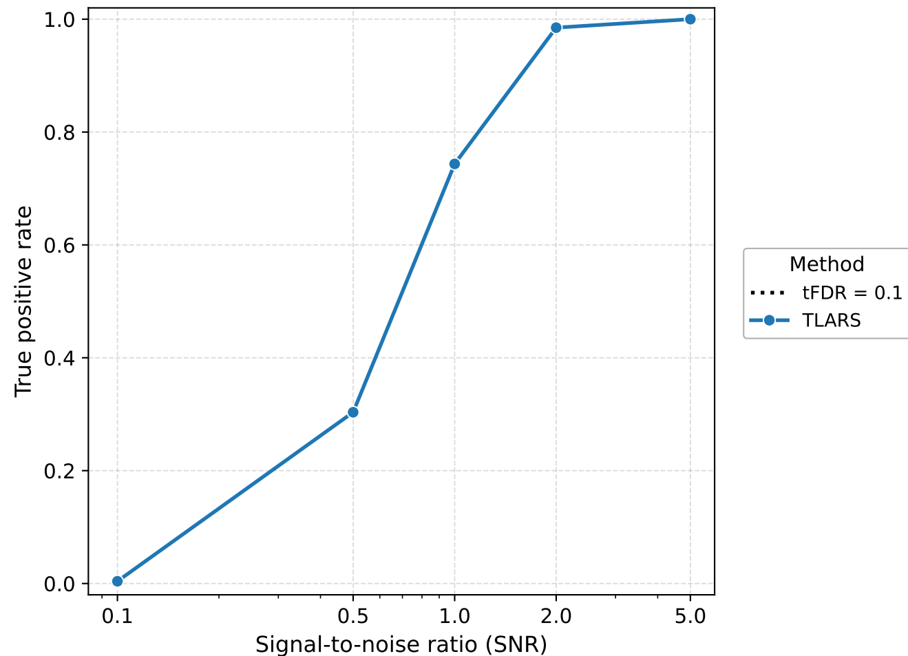
TPR
