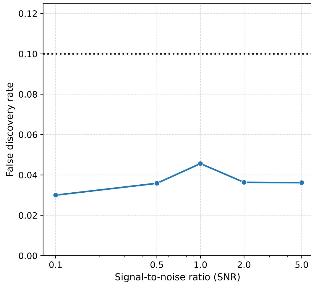
FDR
