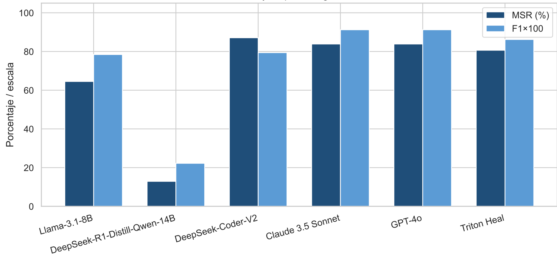
MSR y F1 por configuración
