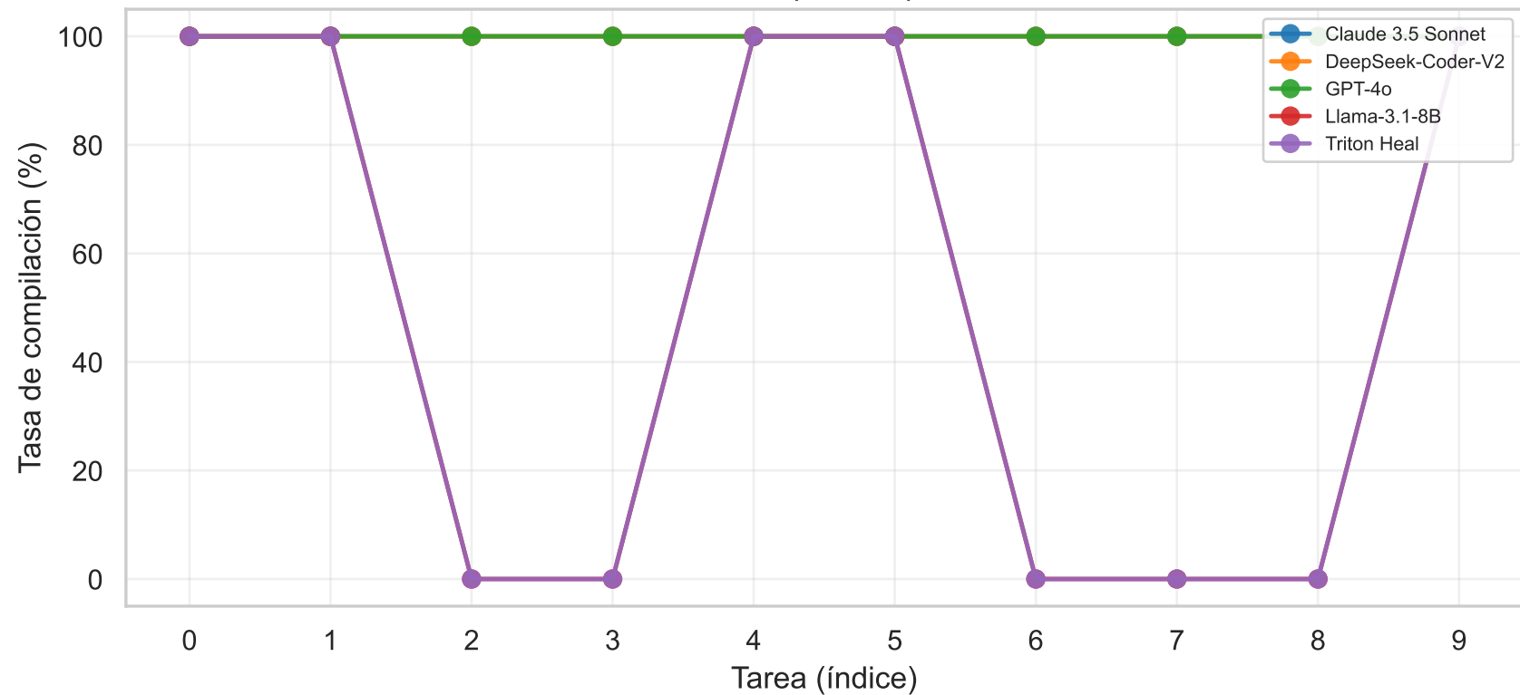
Tasa de compilación por tarea
