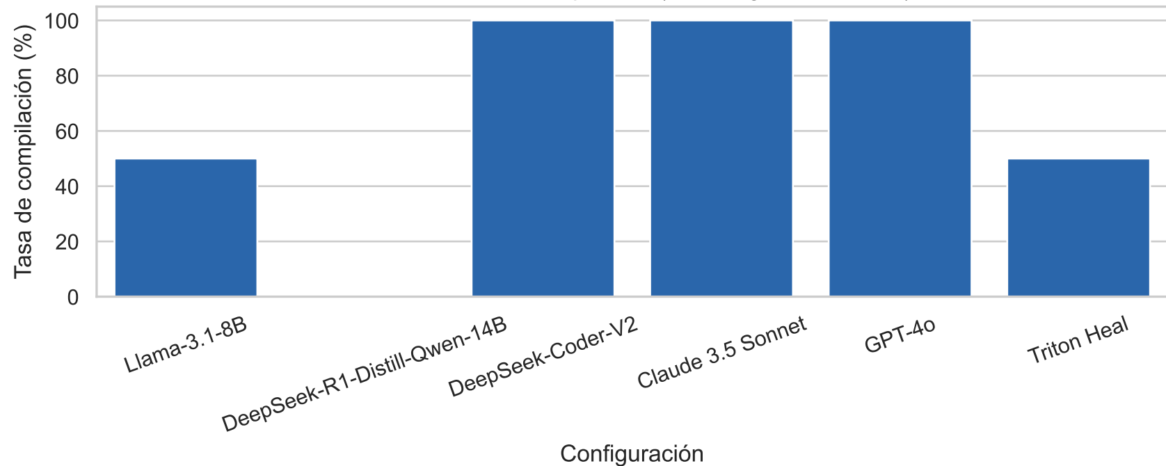
Tasa de éxito de compilación (kernels generados, M4)
