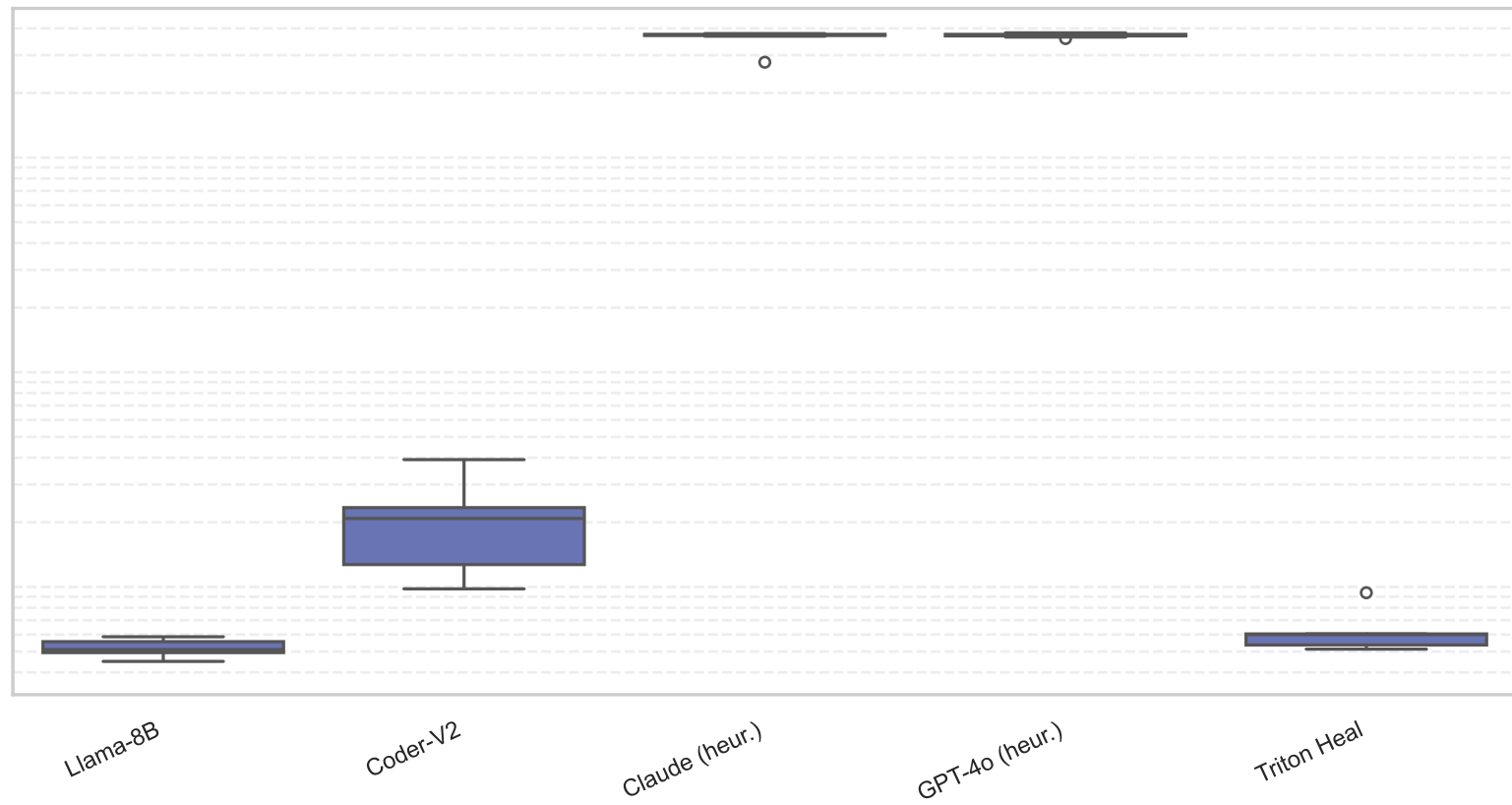
Speedup proxy en tareas con compilación exitosa (M4)
