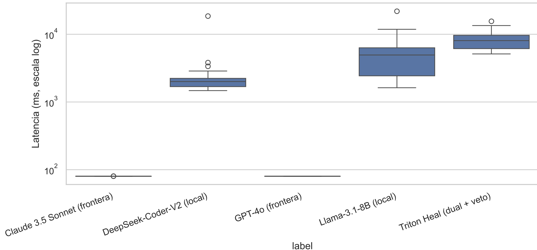
Distribución de latencia de inferencia
