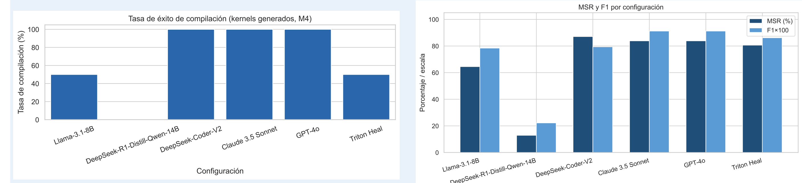
Figure 2: Izq.: tasa de compilación (%) de kernels generados. Der.: MSR (%) y F1×100 en verificación.
