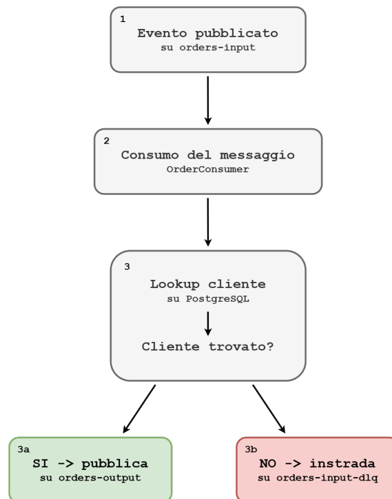
Figura 5.7: Flusso di elaborazione
