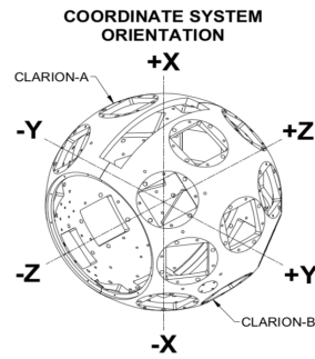
CLARION-B
