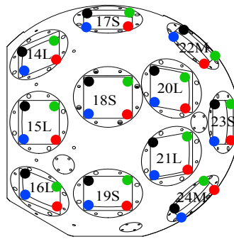
CLARION-B
