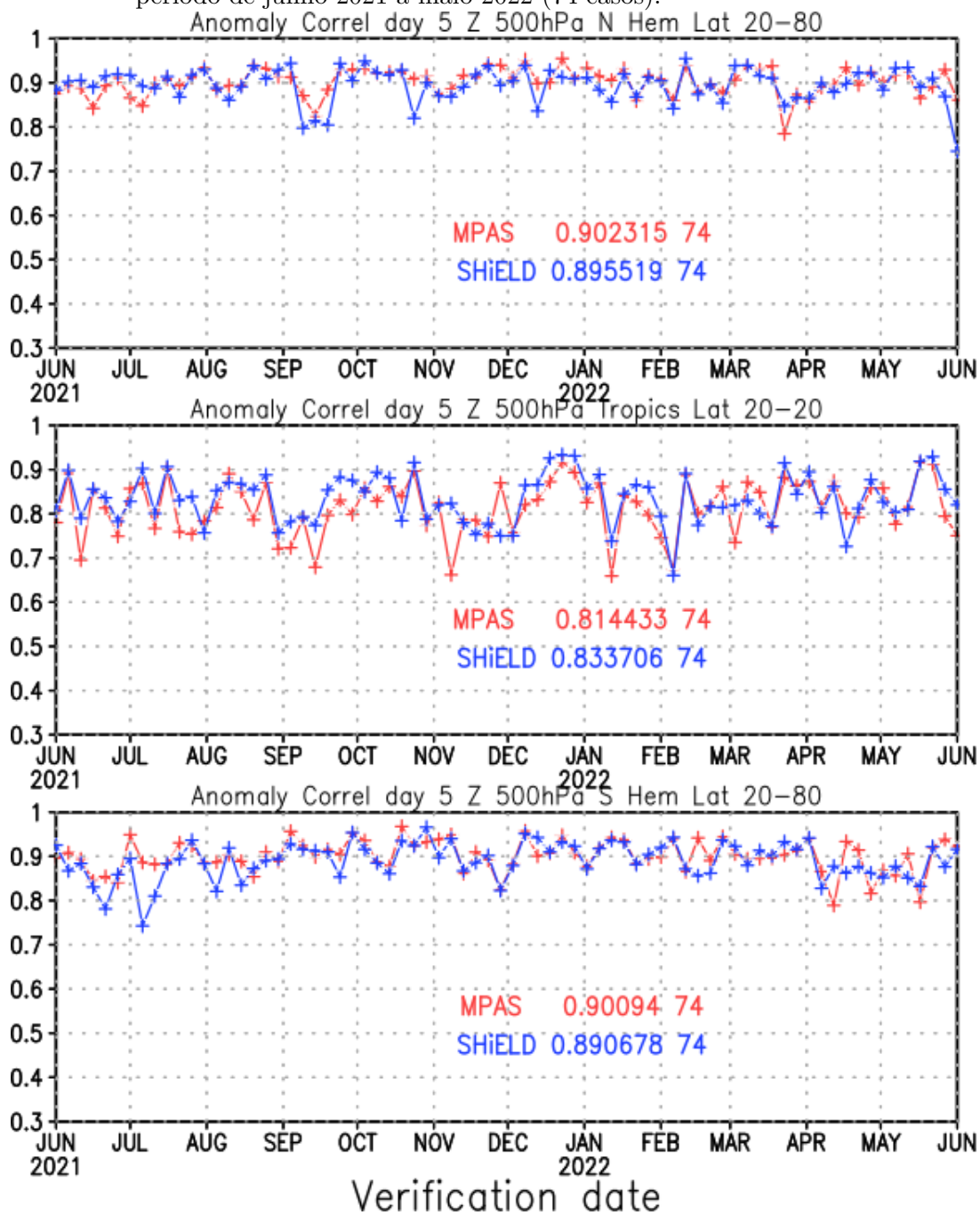
Figura 3.5 - Series temporais da ACC do geopotencial a 500 hPa dos modelos MPAS (vermelho) e SHIELD (azul), para o Hemisfério Norte (painel superior), trópicos (médio) e Hemisfério Sul (painel inferior). Previsões de 120 h (5 dias) para o período de junho 2021 a maio 2022 (74 casos).
