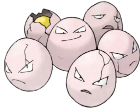
Exeggcute
