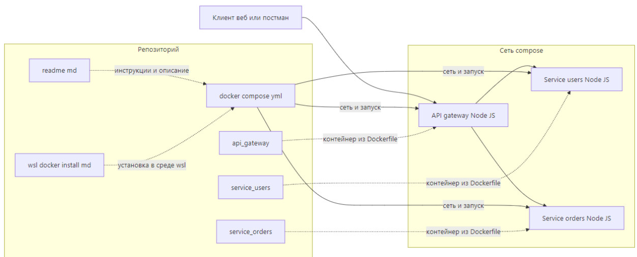
Рис. 1 Схема проекта
