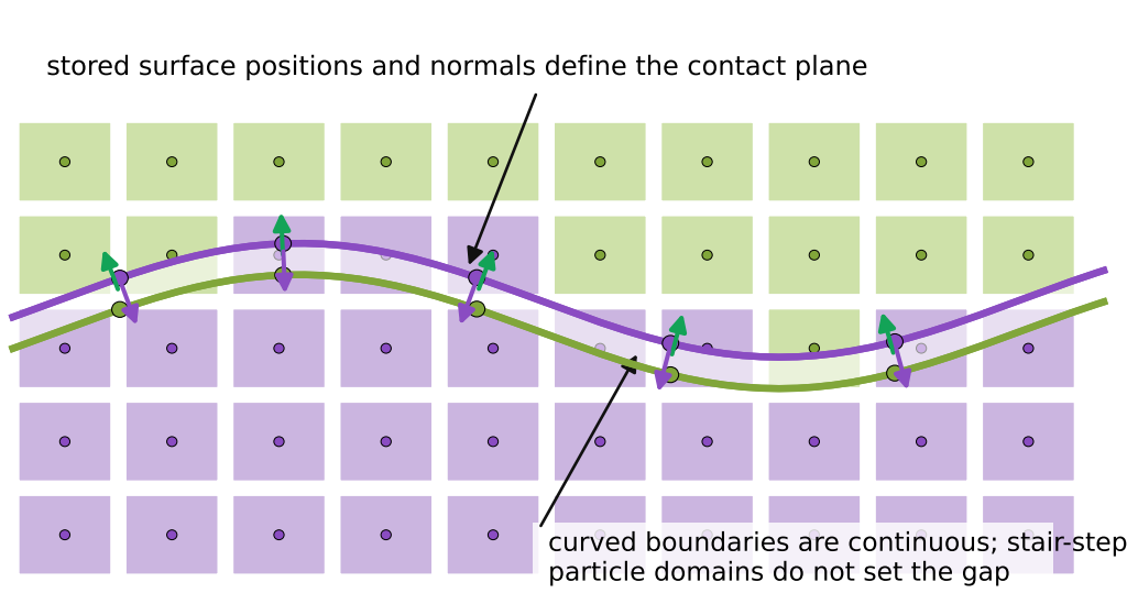
(d) Exact surface contact from cohesive-zone geometry
