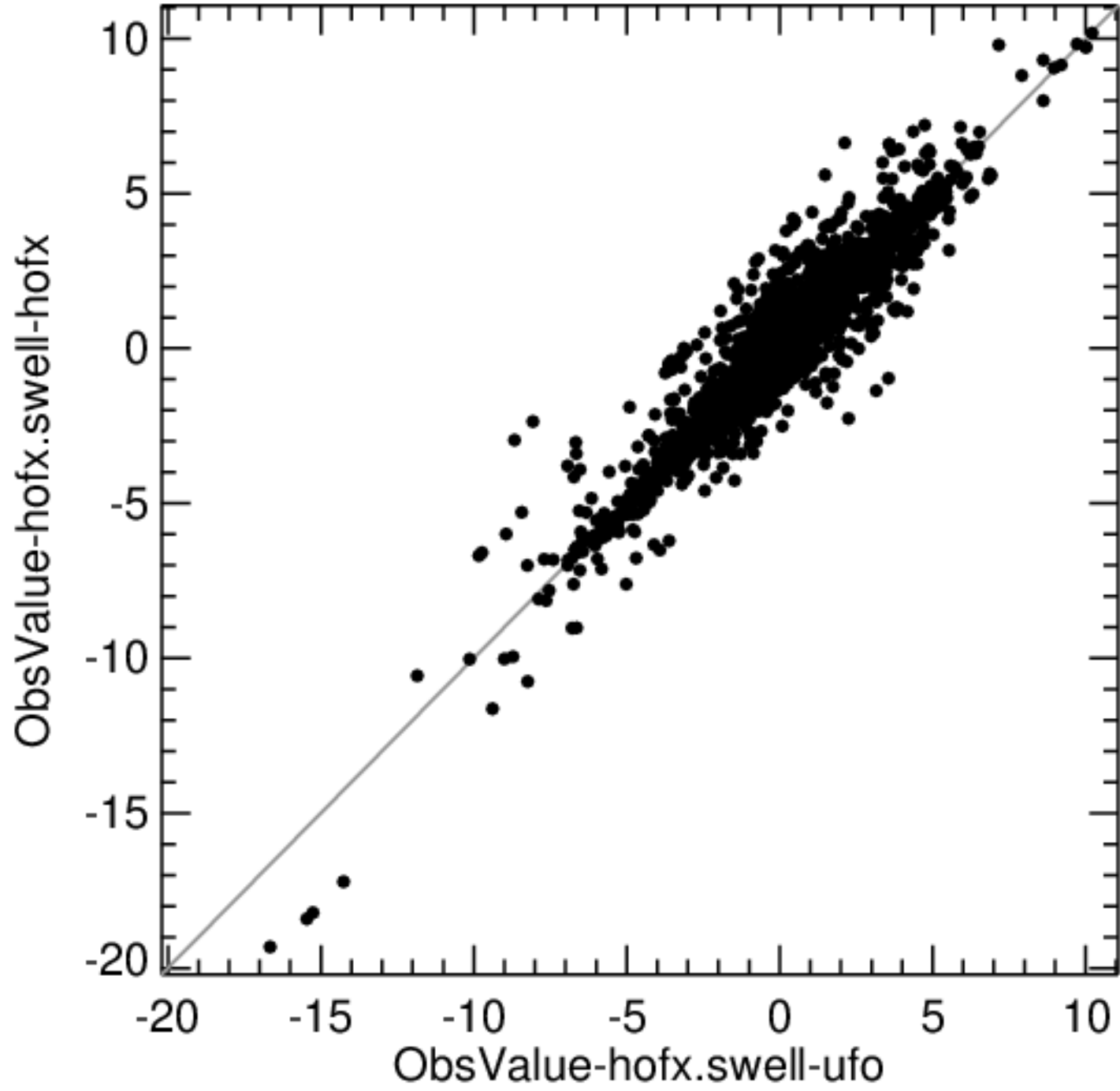
sonde virtualTemperature
