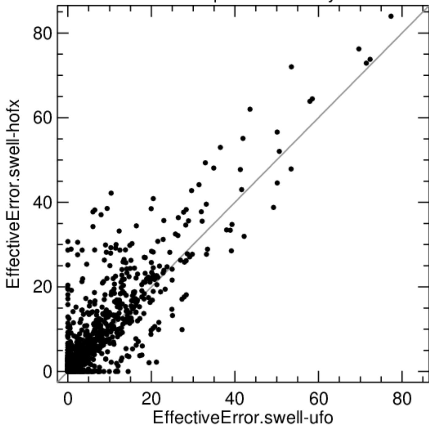
sonde specificHumidity
