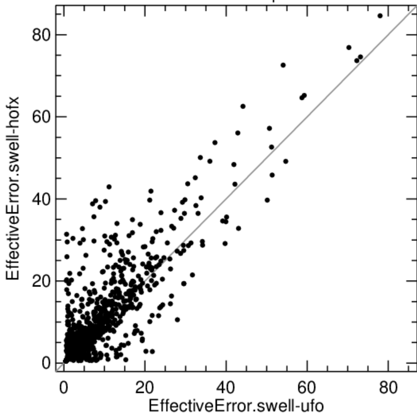
sonde virtualTemperature
