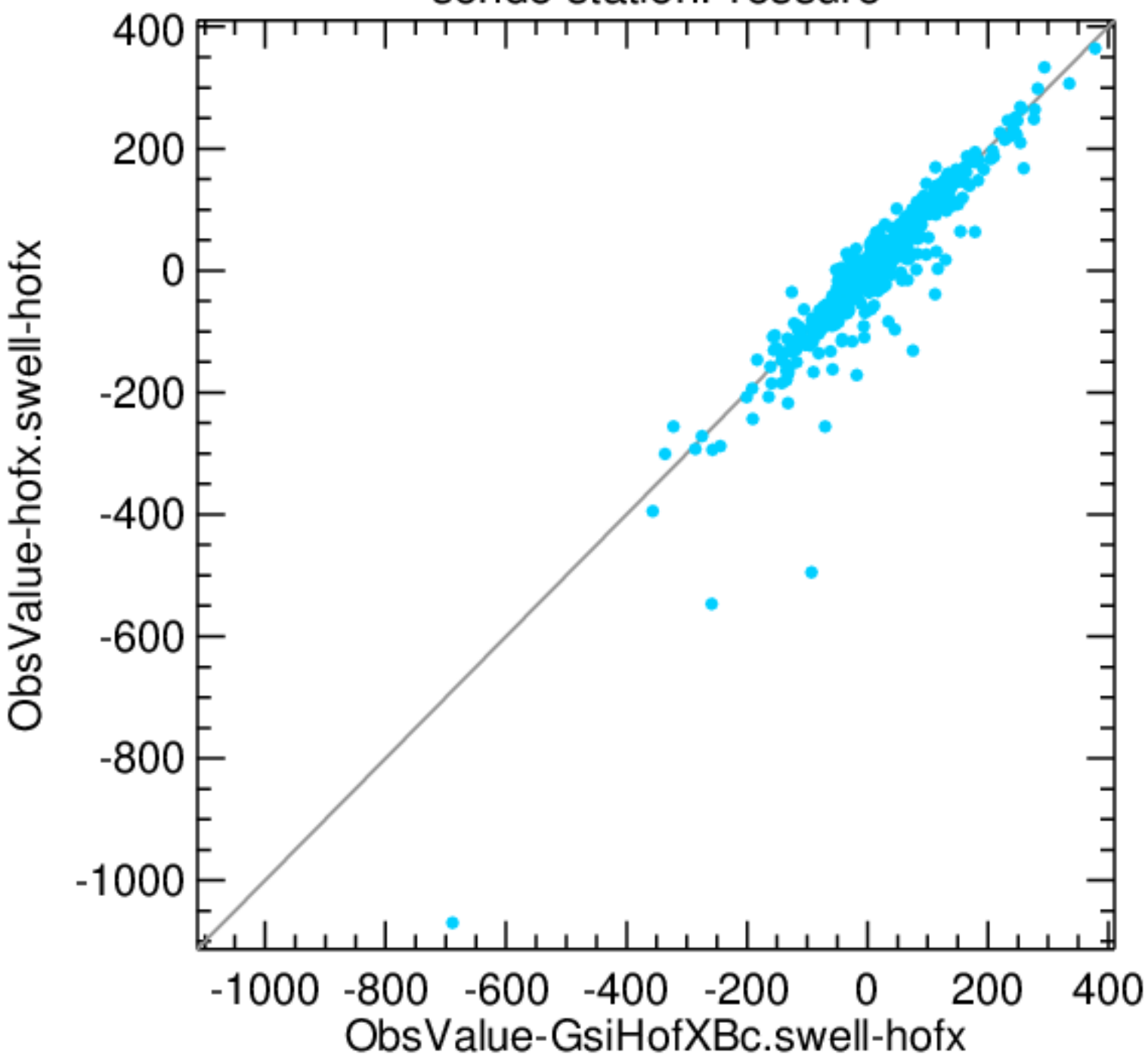
sonde stationPressure
