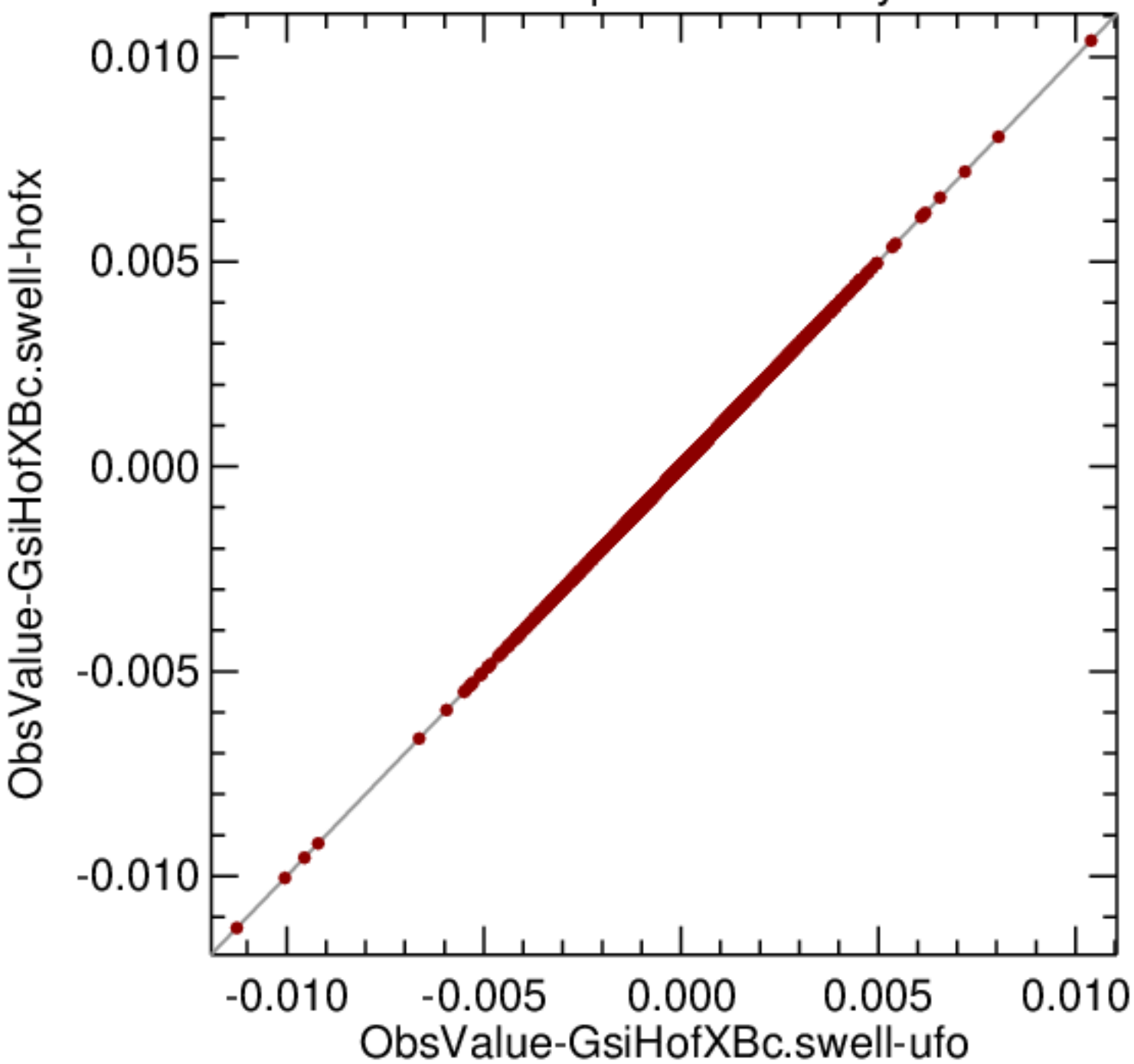
sonde specificHumidity
