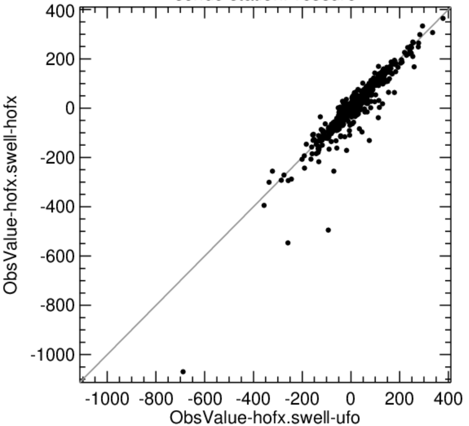
sonde stationPressure
