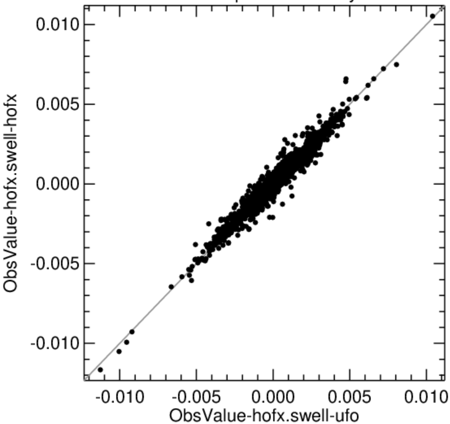
sonde specificHumidity
