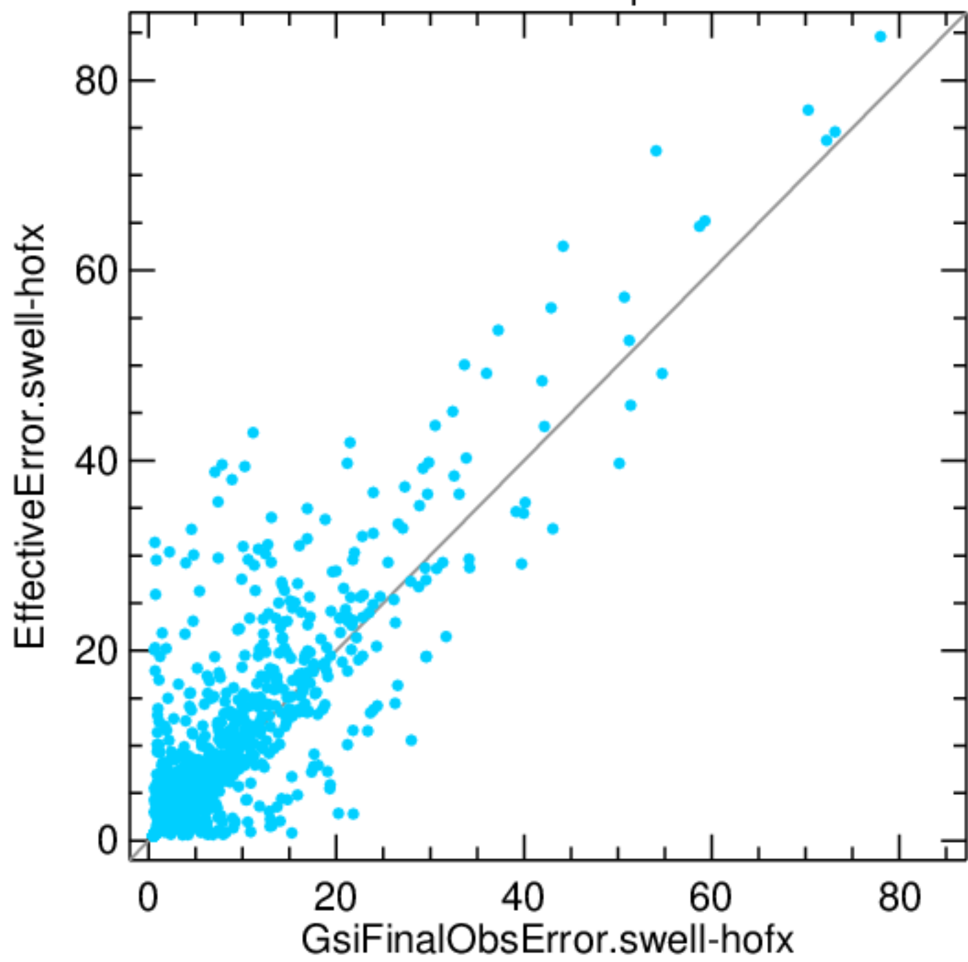
sonde virtualTemperature
