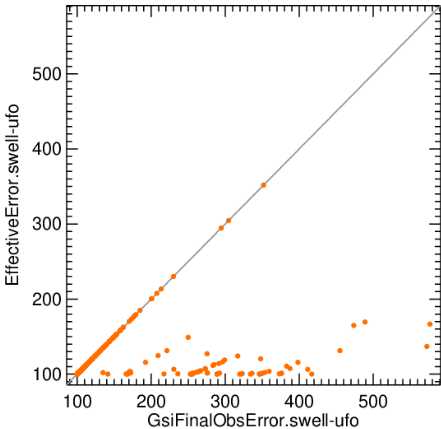
sonde stationPressure
