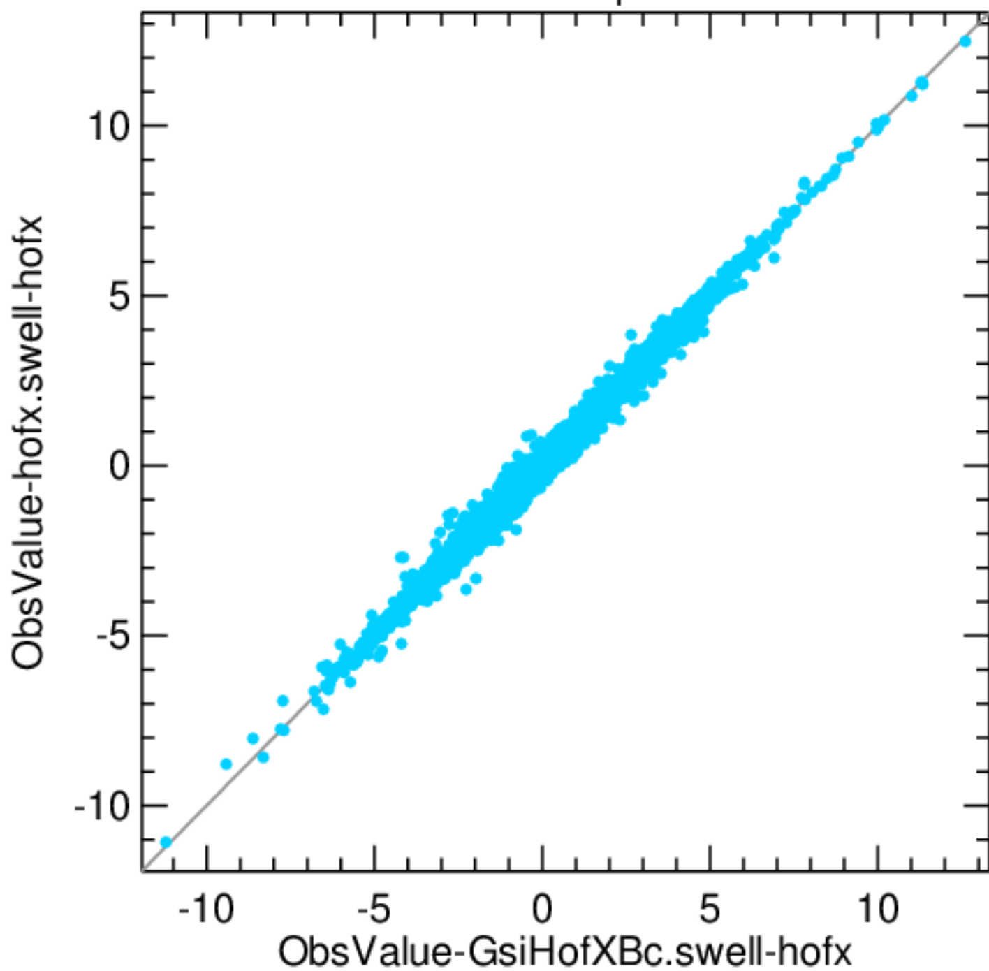
sonde airTemperature
