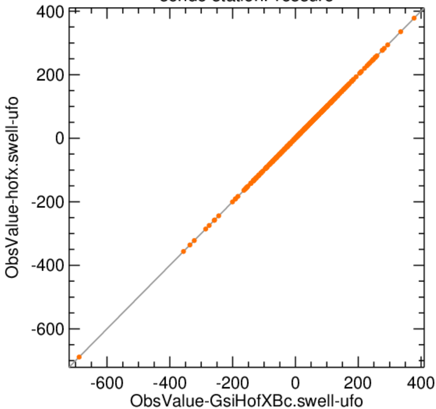
sonde stationPressure
