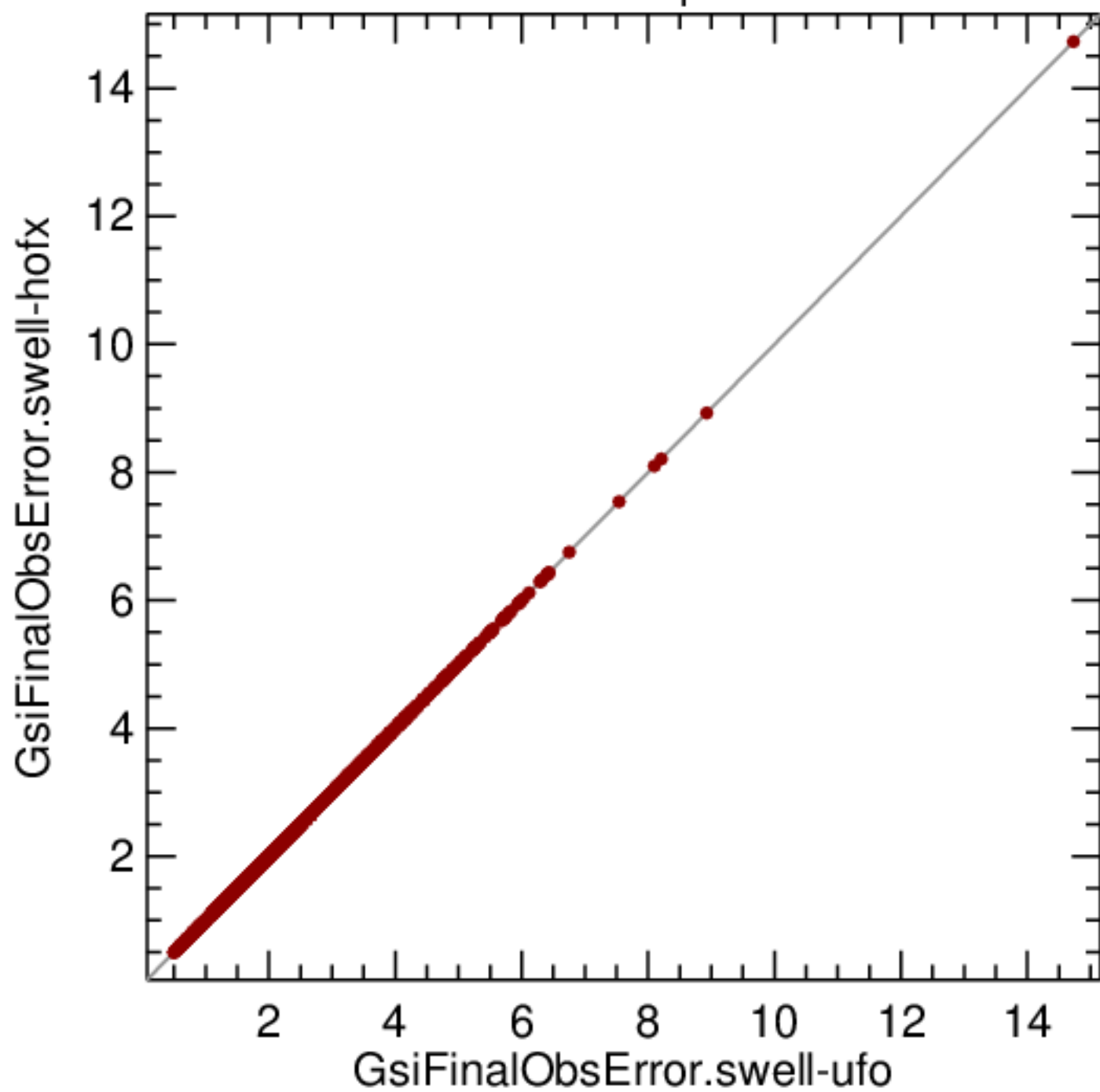
sonde airTemperature
