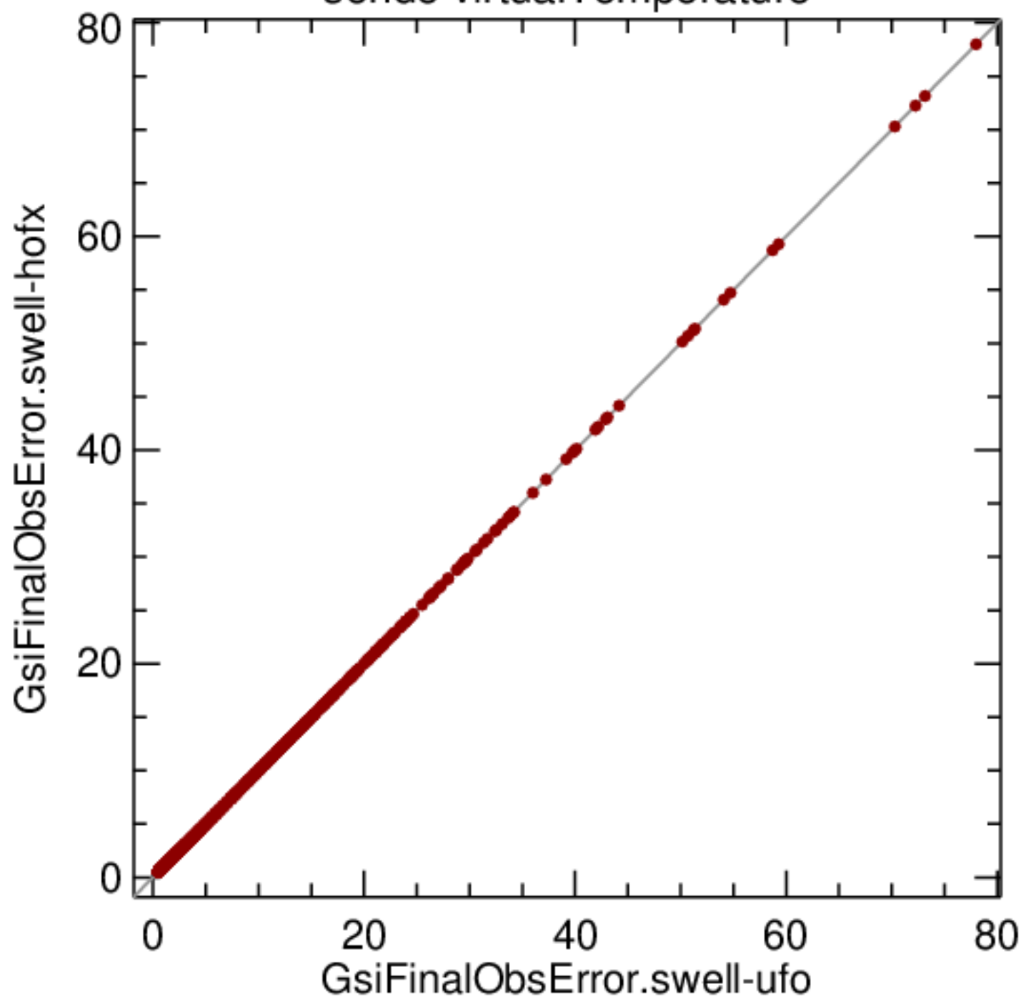
sonde virtualTemperature
