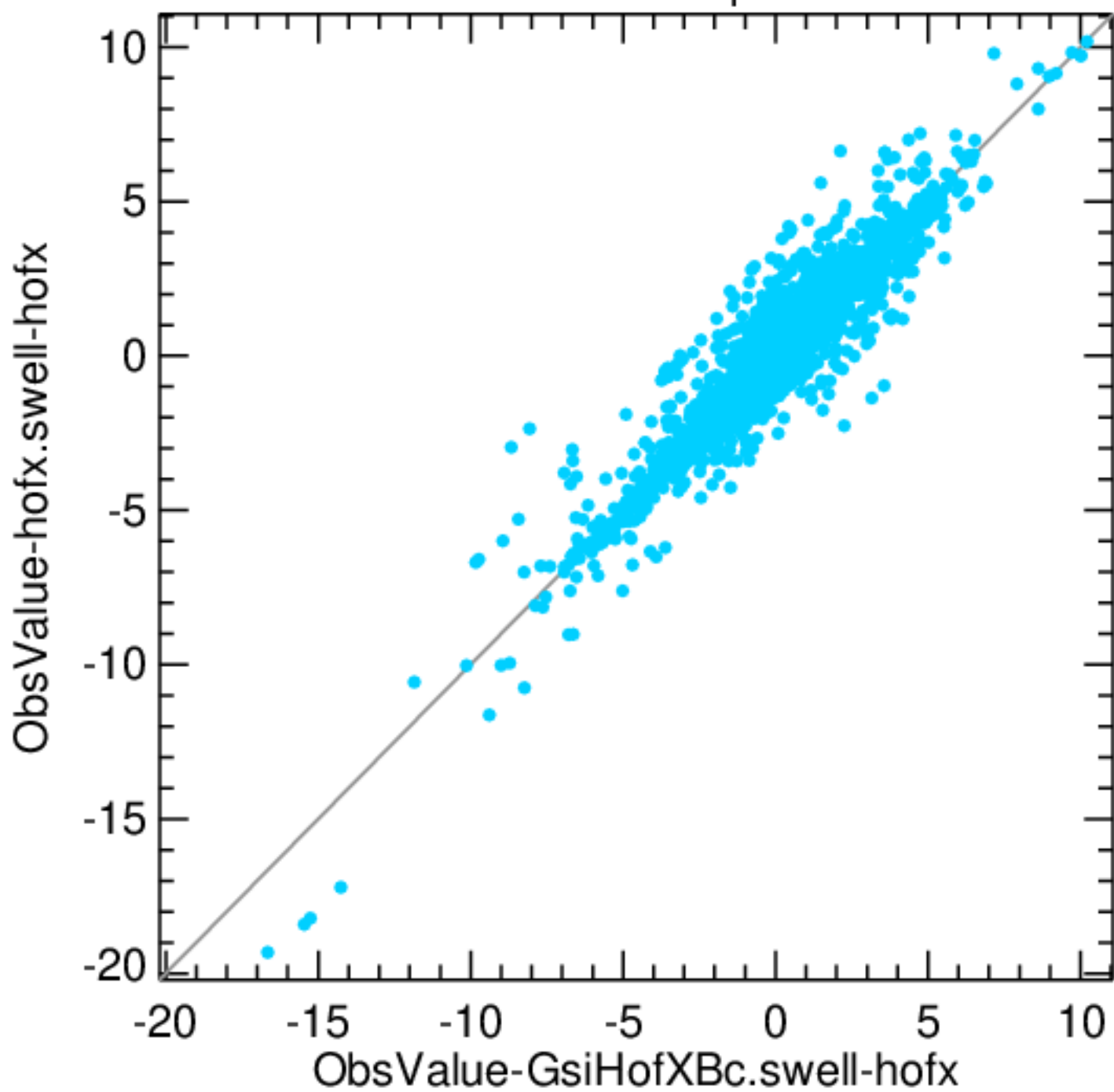
sonde virtualTemperature
