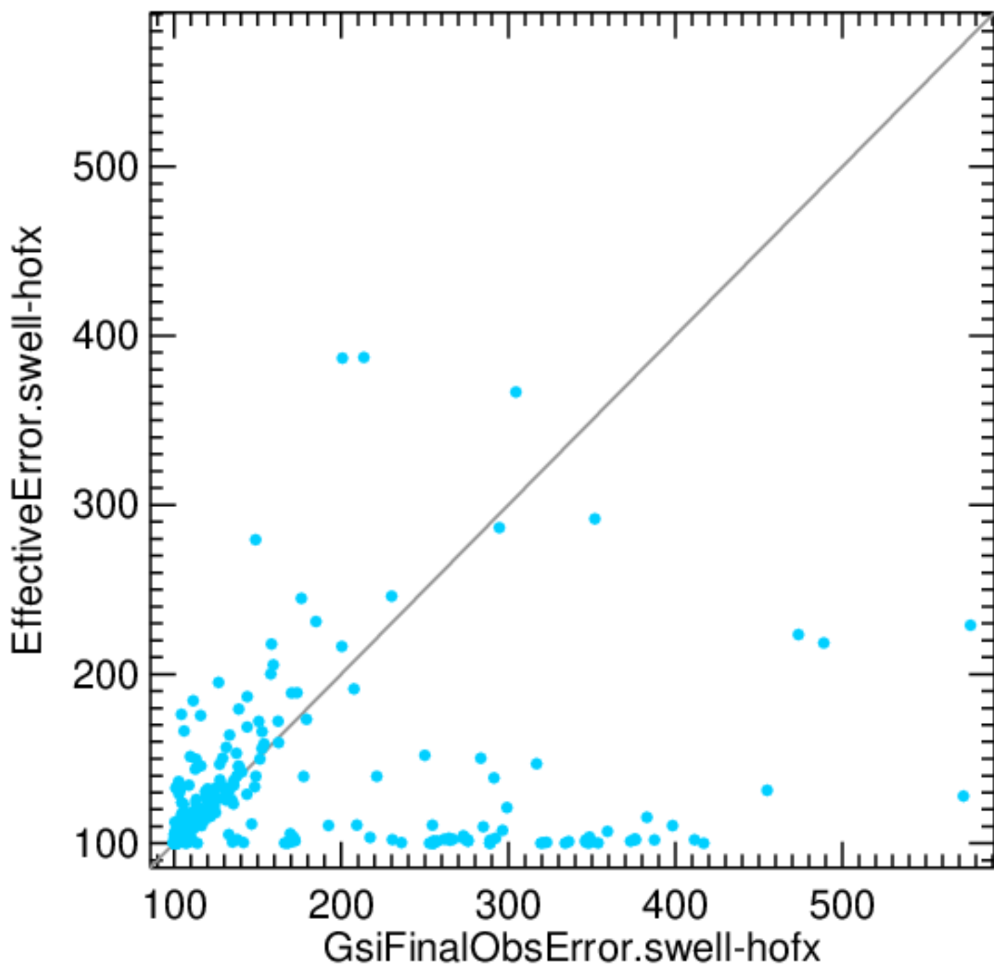
sonde stationPressure
