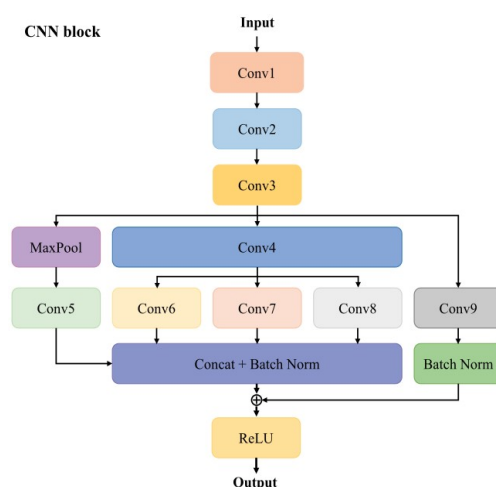
شکل ۱۳-۳: ساختمان CNN Block
