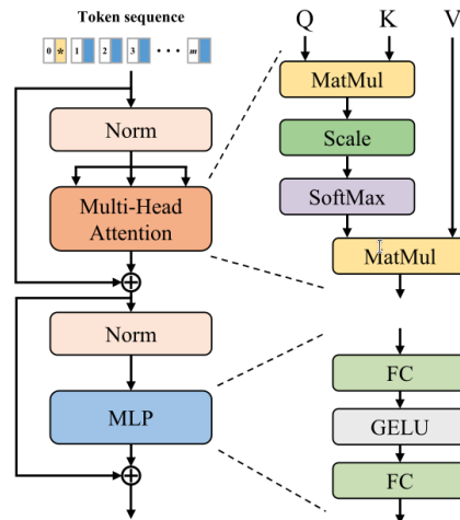
شکل ۳-۱۴: transformer encoder.
