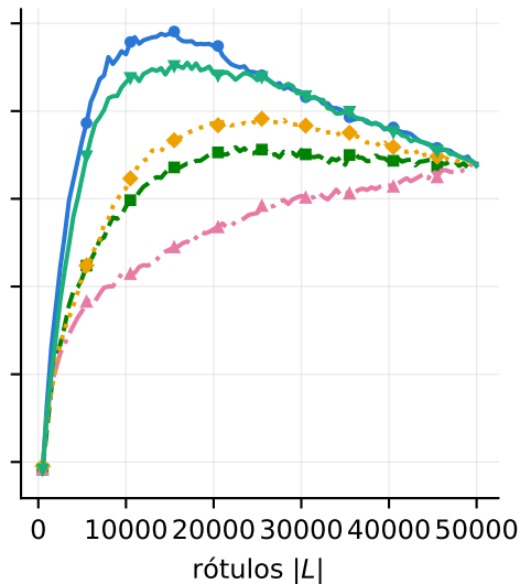
SGD logístico
