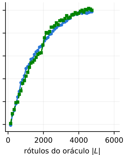
SGD logístico
