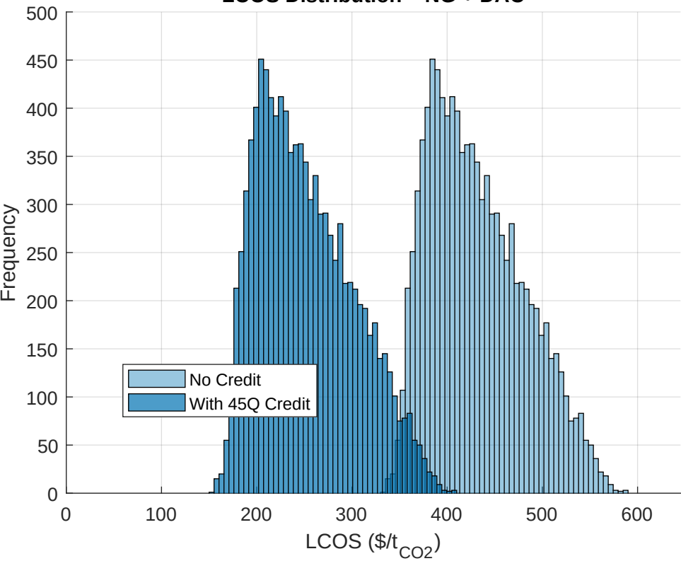
LCOS Distribution - NG + DAC
