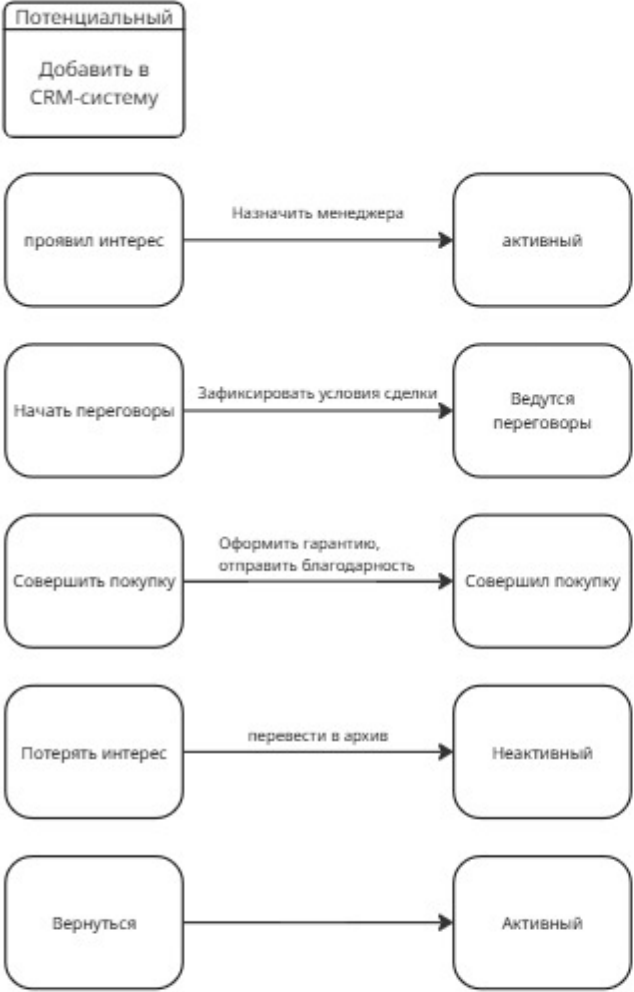
Диаграмма состояний для объекта Клиент
