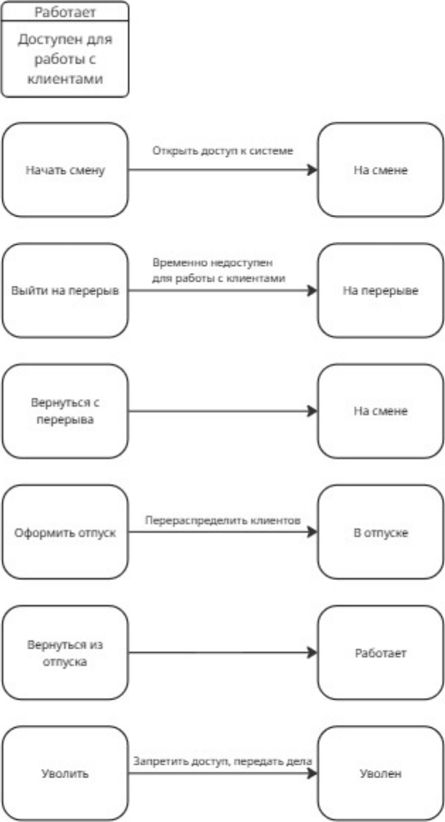
Диаграмма состояний для объекта Сотрудник
