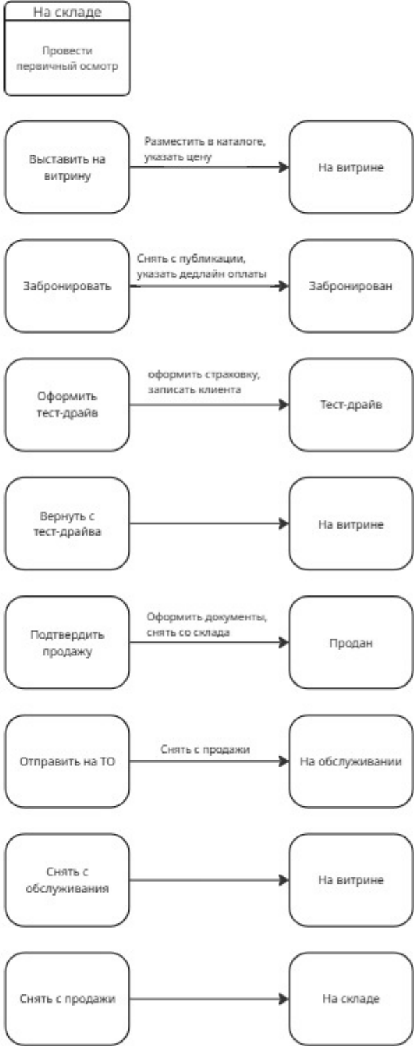
Диаграмма состояний для объекта Автомобиль
