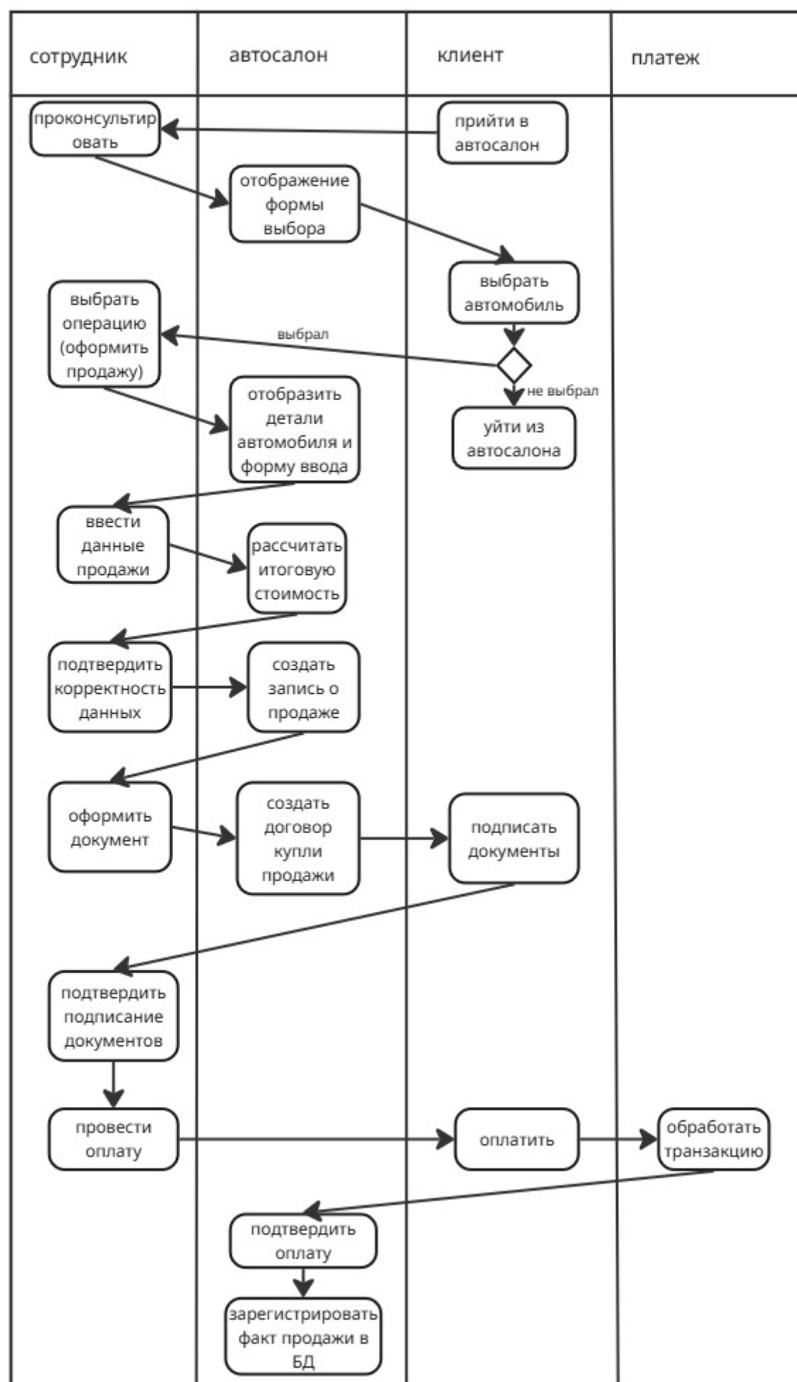
диаграмма деятельности
