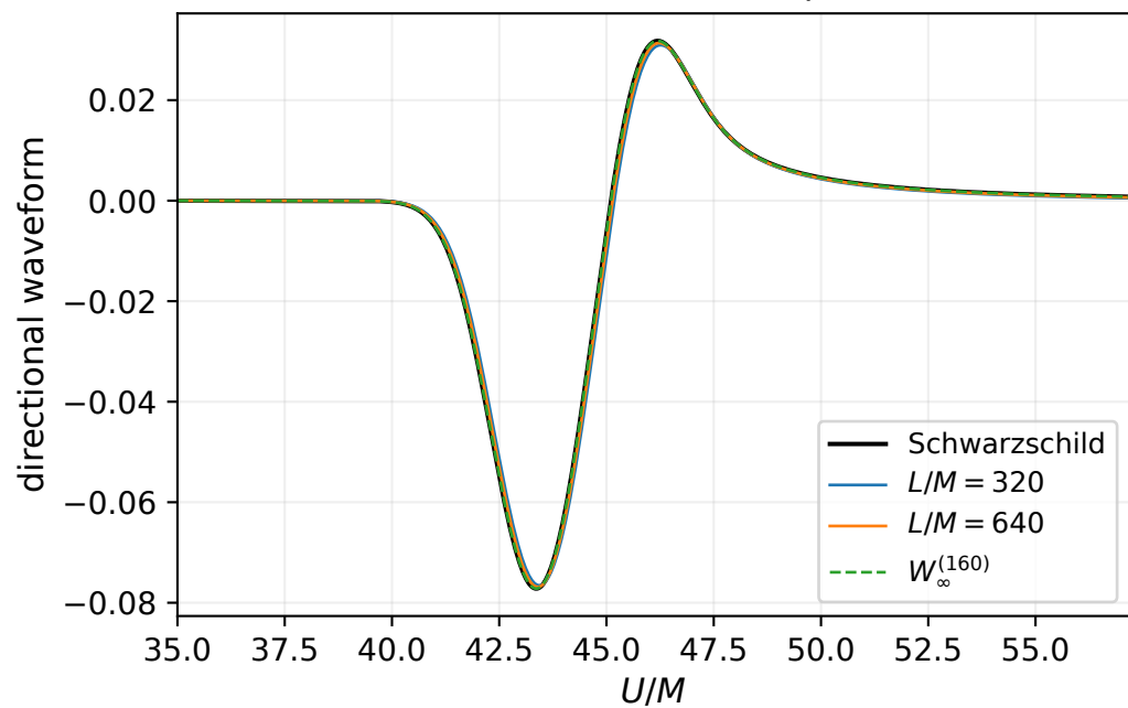
(d) Caustic direction, \gamma = \pi
