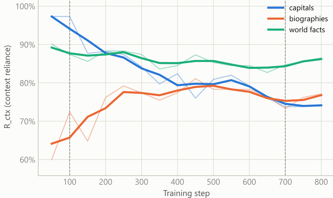
Alpaca SFT
