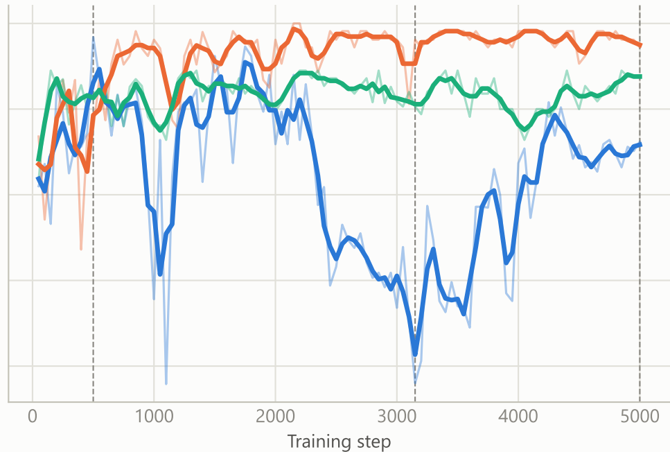
Tulu SFT
