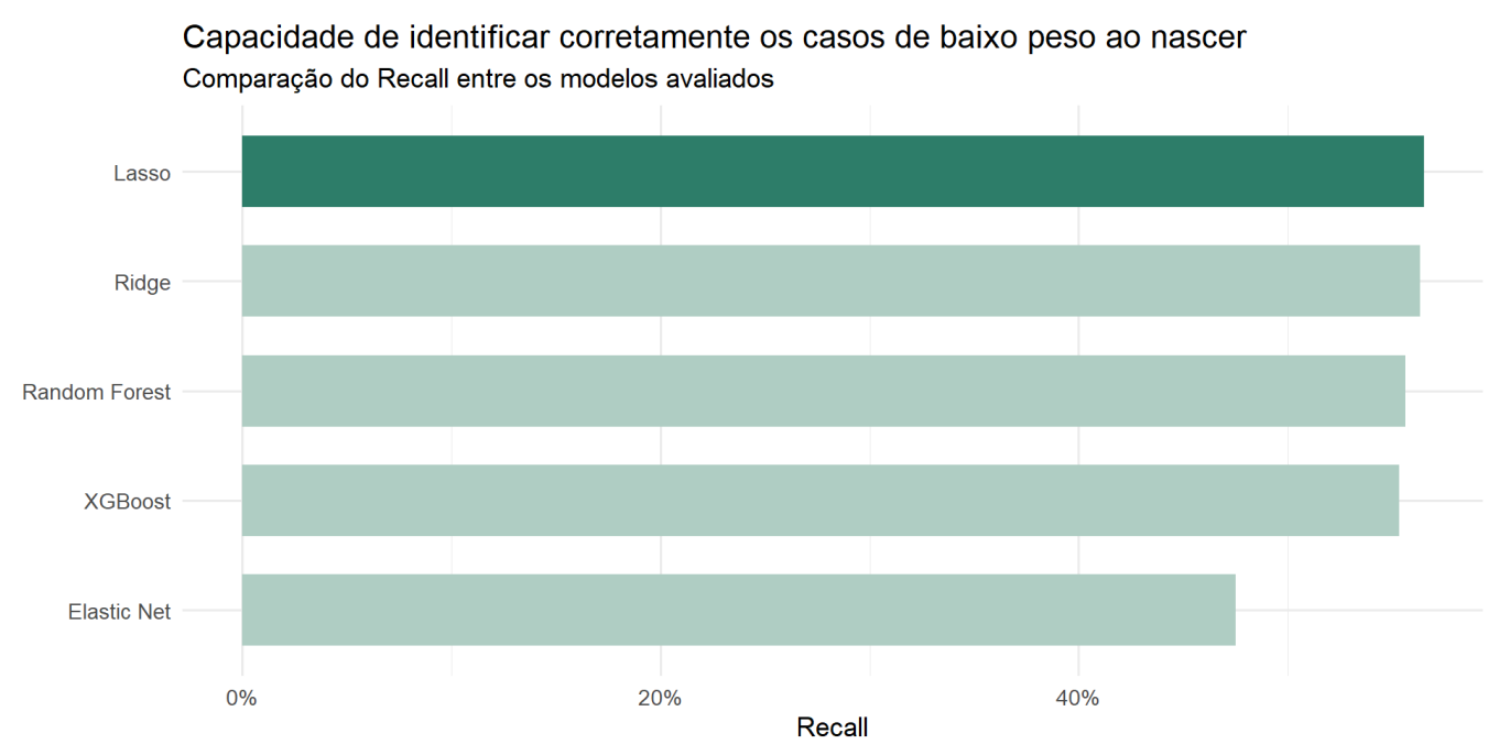
Figura 4. Comparação da capacidade de identificação correta dos recém-nascidos com baixo peso ao nascer (Recall).
