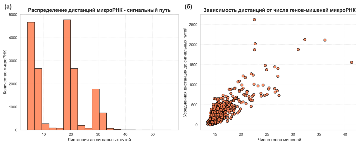
Рис. 1: Распределение микроРНК по среднему расстоянию до рассматриваемых сигнальных путей
