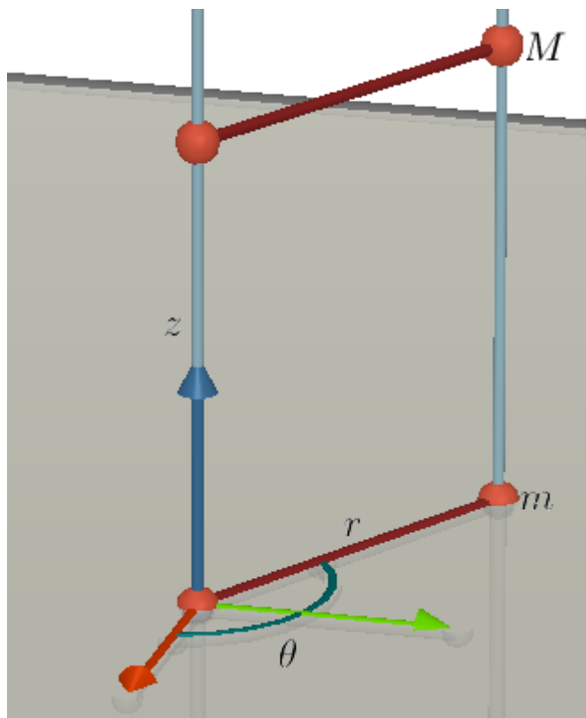
FIGURE 1.5 – Coordonnées cylindriques
