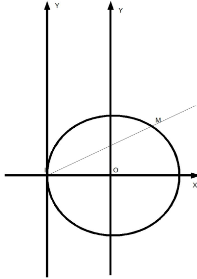
FIGURE 5.1 – Représentation paramétrique rationnelle
