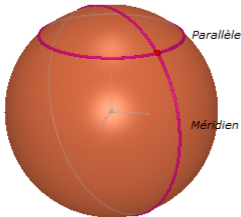
FIGURE 1.7 – Méridiens-Parallèles
