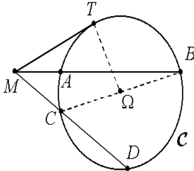
FIGURE 5.6 – Puissance d'un point par rapport à un cercle
