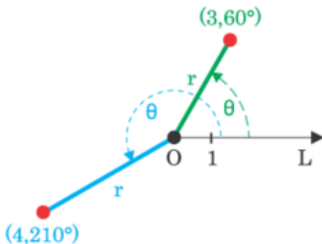
FIGURE 1.2 – Exemple de coordonnées polaires
