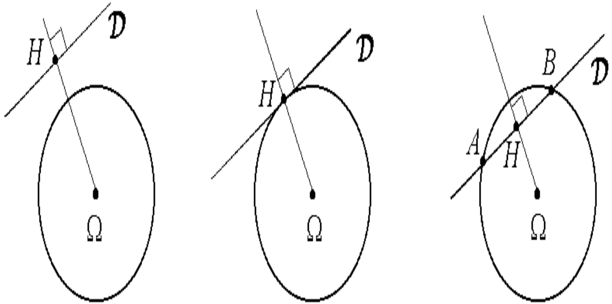
FIGURE 5.3 – Intersection de cercle et droites
