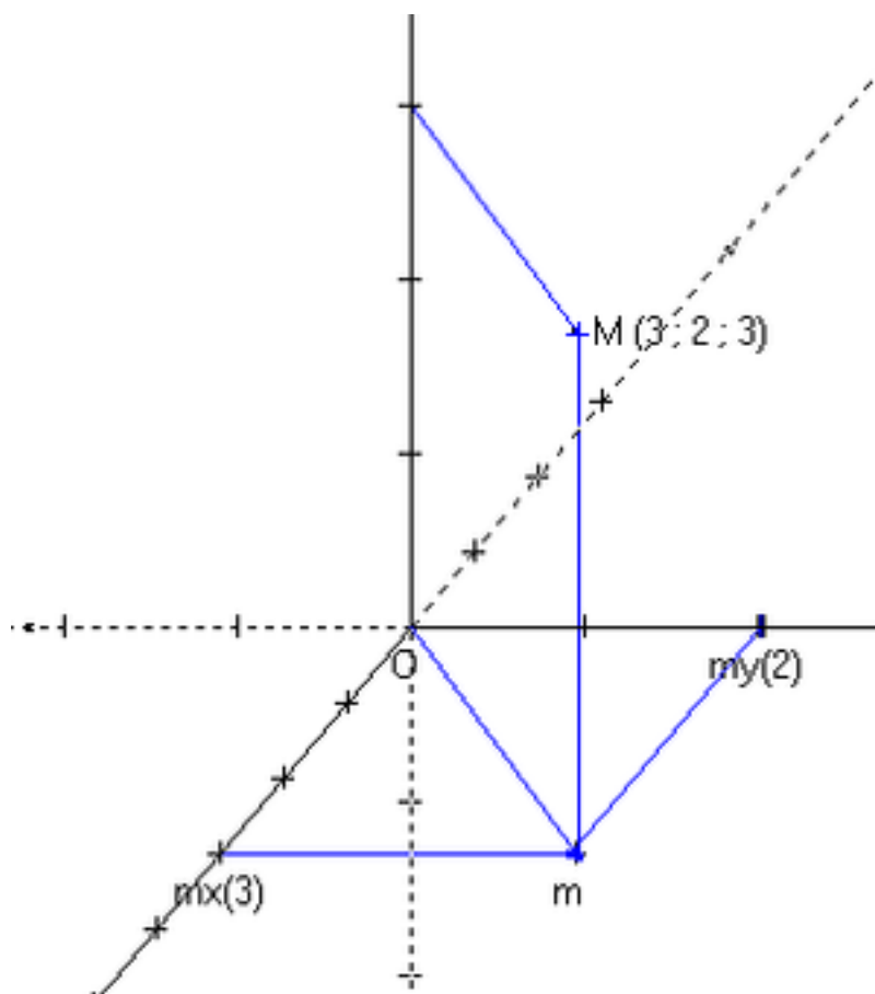
FIGURE 1.4 – exemple de coordonnées cartésiennes
