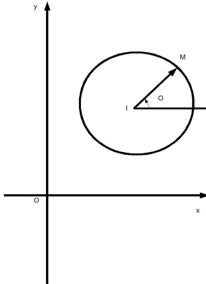
FIGURE 5.2 – Représentation paramétrique
