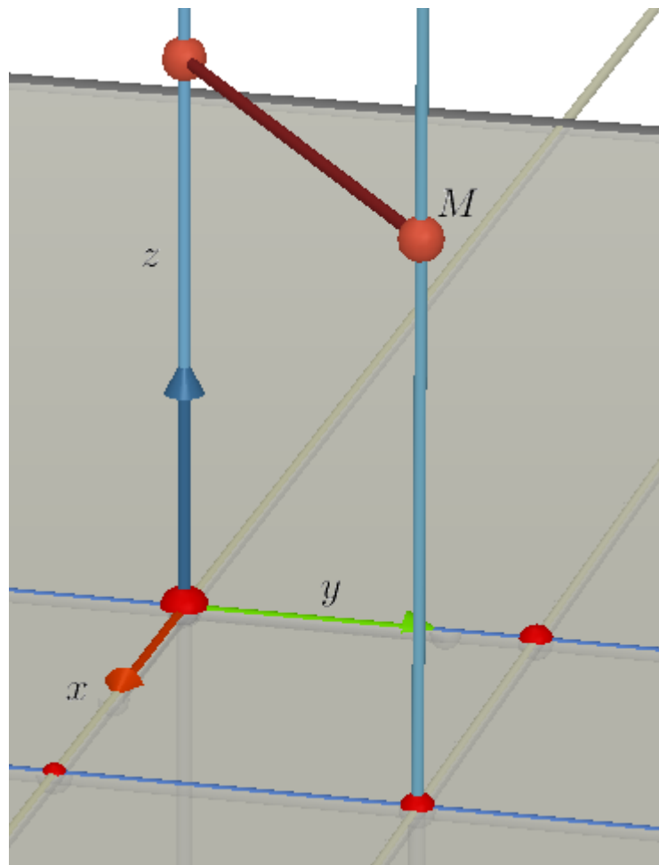
FIGURE 1.3 – Coordonnées cartésiennes
