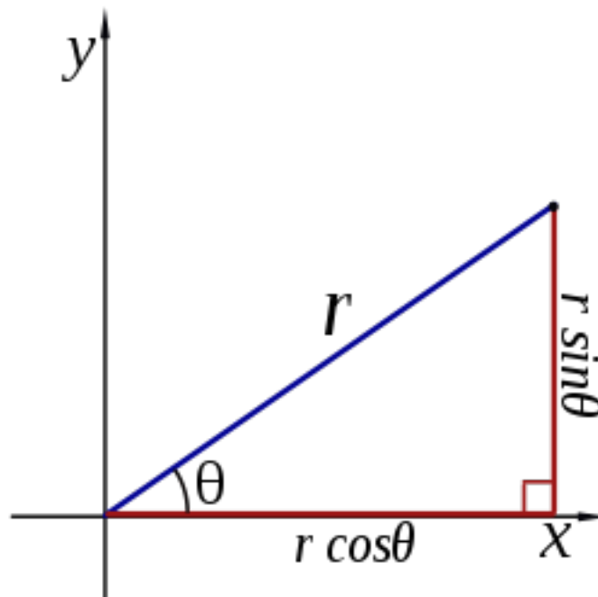
FIGURE 1.1 – Exemple de coordonnées polaires
