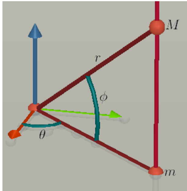
FIGURE 1.6 – Coordonnées sphériques
