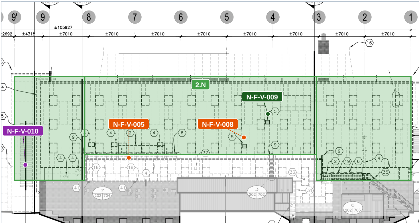
Élévation nord, axes 9 à 1
