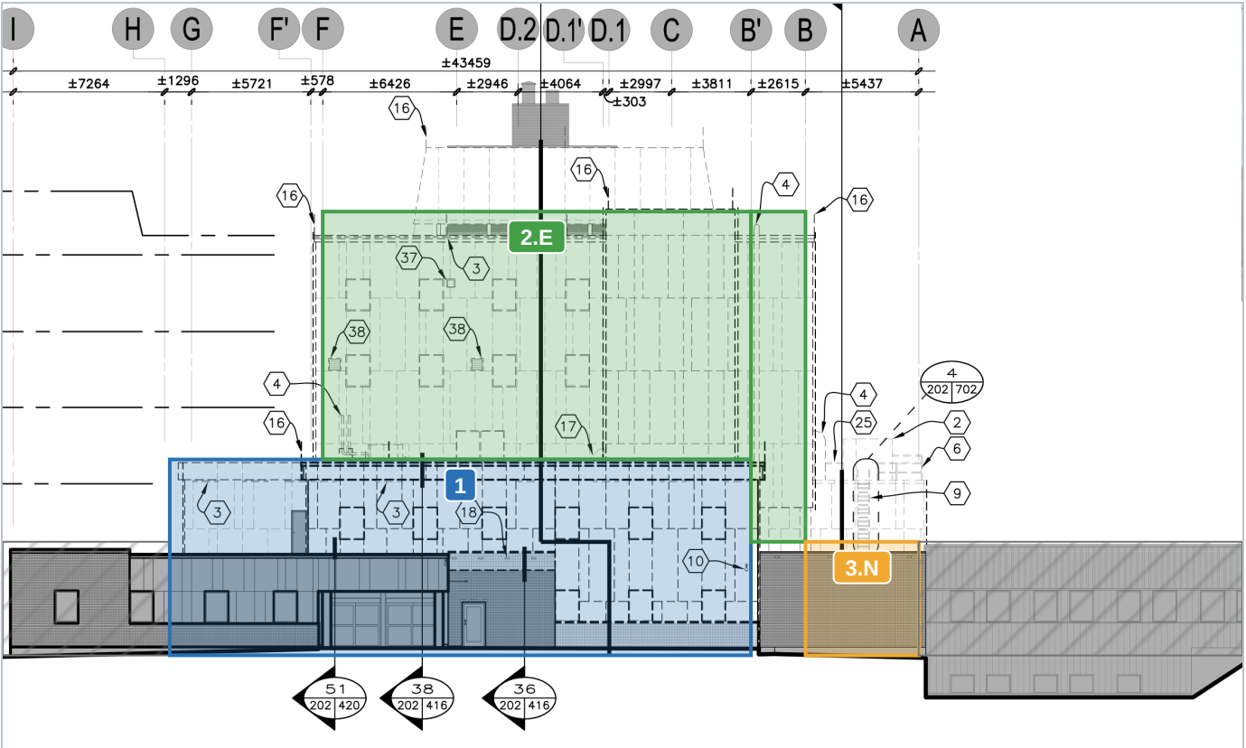
Élévation est (G) — le sud à gauche, le nord à droite.
