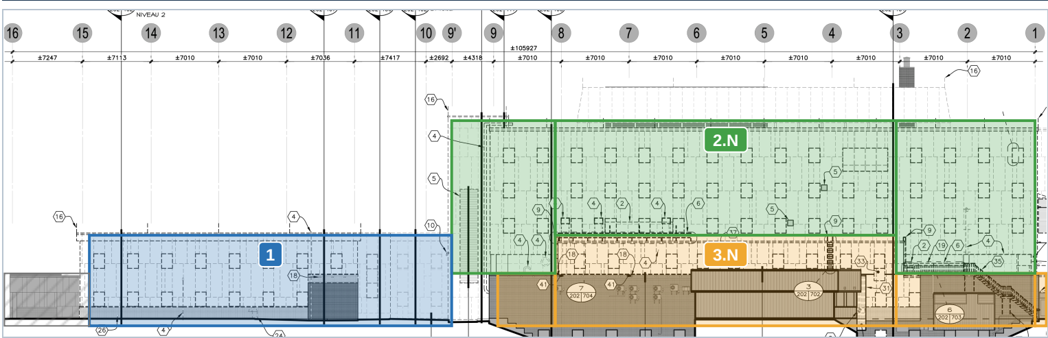
Élévation nord (F) — l'est à gauche, l'ouest à droite.
