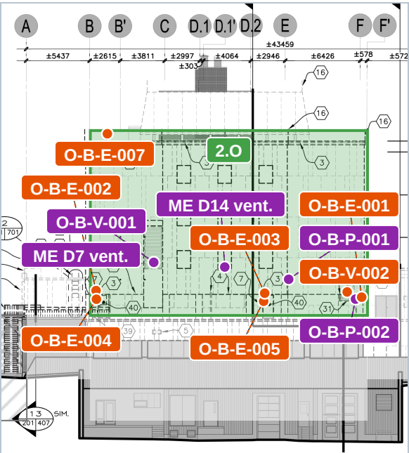
Ouest, axes A à F'
