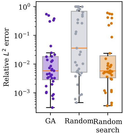
Pendulum
