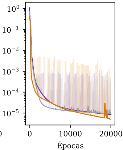
Condução de calor (rodada 32)
