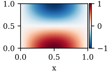
PINN (AG), rodada 0, L^2 = 9,02\text{e-}3
