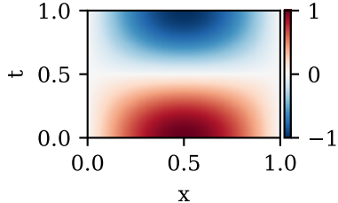
Corda vibrante: Exata
