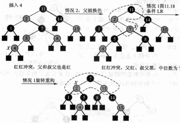
图 11.20 红黑树插入示例
