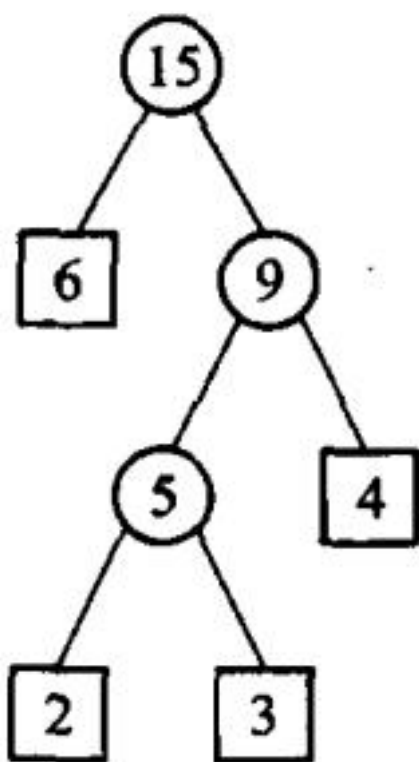
图 5.19 Huffman 树的构造过程
