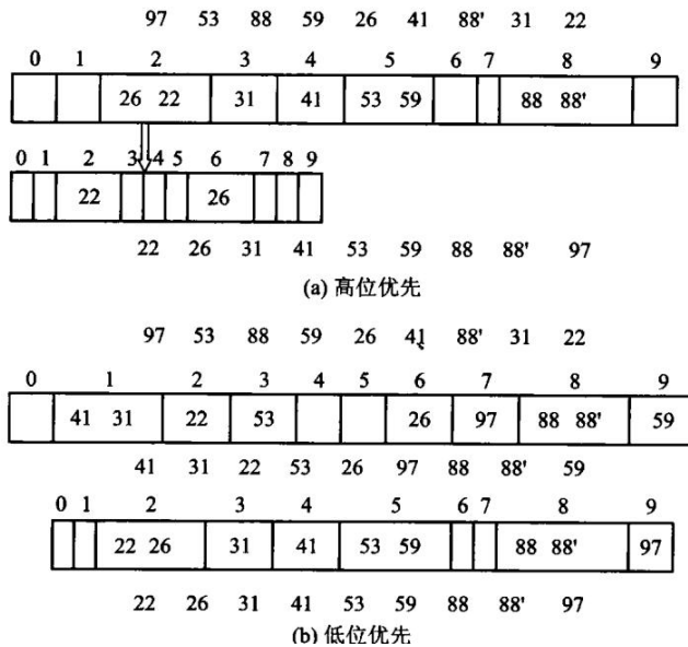
(b) 低位优先; 图 8.10 基数排序
