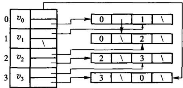
图 7.15 有向图的十字链表示例
