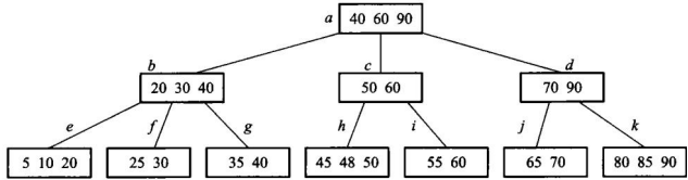
图 11.11 从图 11.9 的 3 阶 B + 树中删除 75 后
