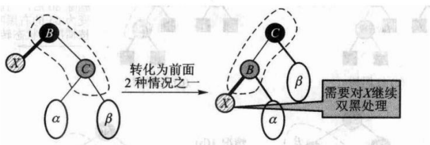
图 11.24 情况 3 双黑的兄弟结点为红色
