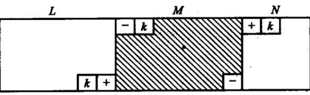
图 12.13 把块 M 释放回可利用空间表
