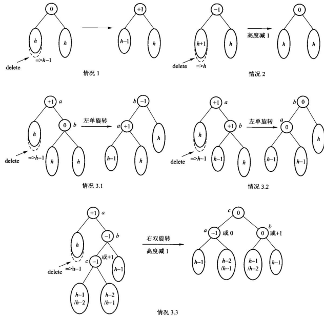
图 12.35 AVL 树删除之后的平衡操作
