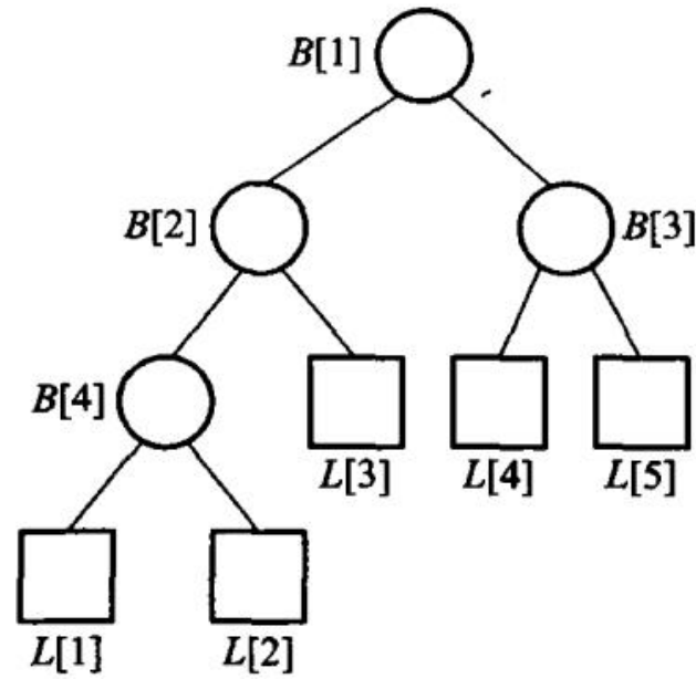
图 9.4 含有 5 个选手的赢家树
