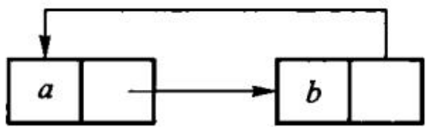
图 12.14 无用单元循环引用
