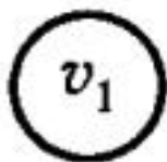
(b) 有向图 G_2 的若干子图；图 7.4 图 7.2 的若干子图
