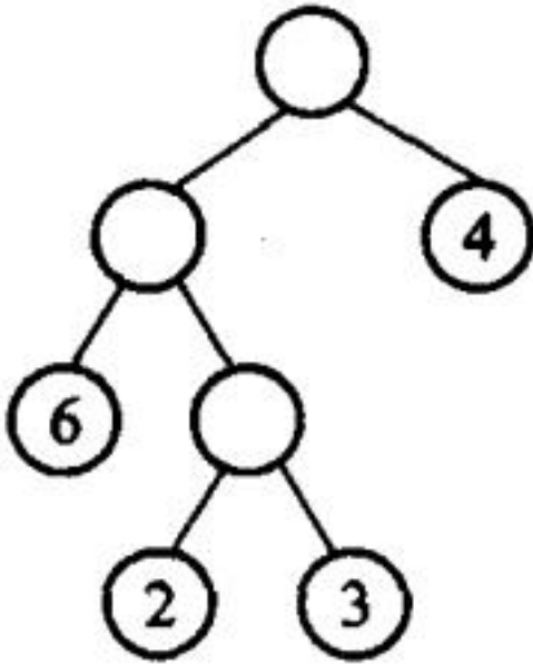
(b) 外部路径为 31
