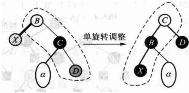
图 11.21 情况 1(a):
