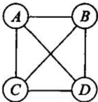
(a) 无向完全图
