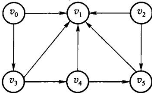
(a) 有向图
