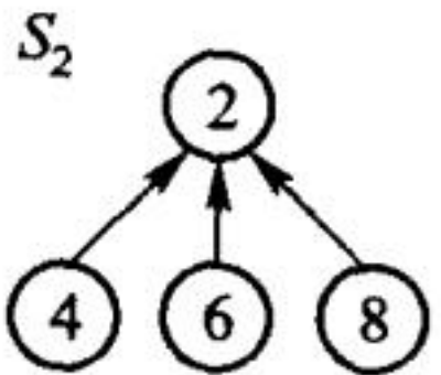
(b) 子集 s_2
