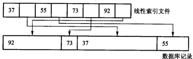
图 11.1 线性索引，图中的数据库记录不等长
