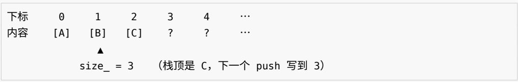
图 3.2 顺序栈：下标 0 是栈底，size_ 是元素个数，也是下一个空位。
