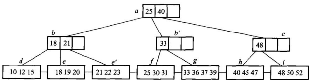
图 11.12 混合型 B+ 树, 内部结点阶为 4, 叶结点阶 5
