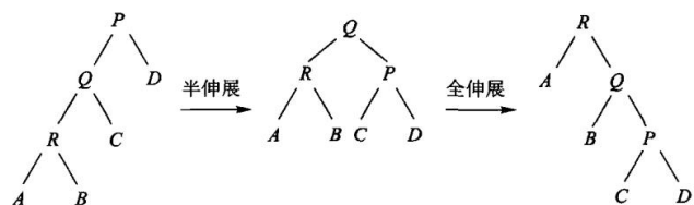
图 12.42 半伸展和全伸展的区别
