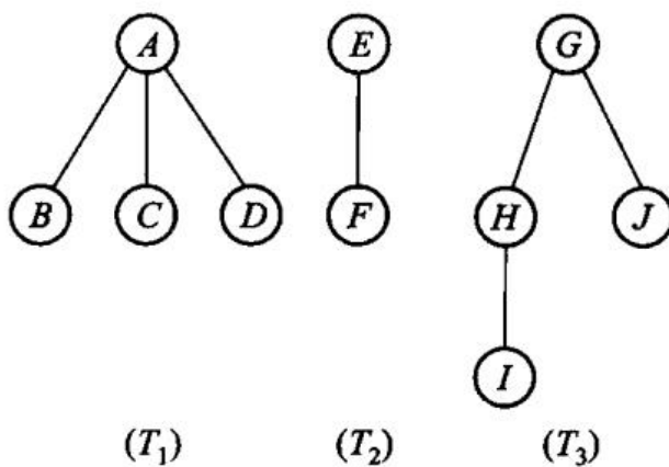
(b) 森林
