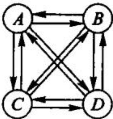
(b) 有向完全图；图 7.3 完全图
