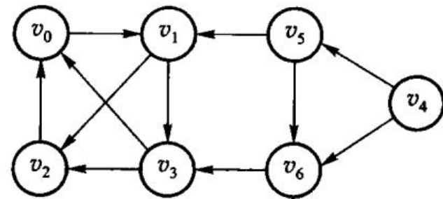
图 7.16 有向图 G
