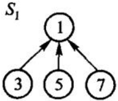
(a) 子集 s_1
