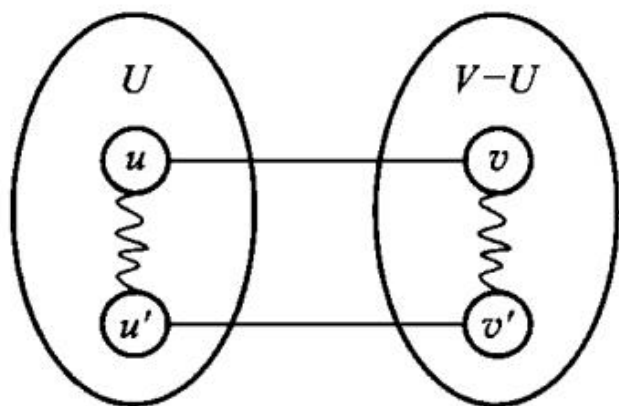
图 7.22 含 (u,v) 的回路
