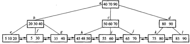
图 11.9 3 阶 B + 树
