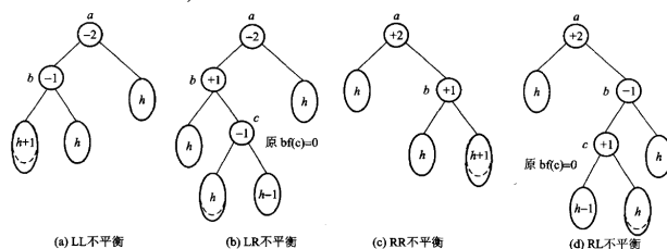
图 12.31 AVL 树的四种失衡类型：(a) LL、(b) LR、(c) RR、(d) RL。圆圈是结点，椭圆是子树，里面的符号是它的高度。
