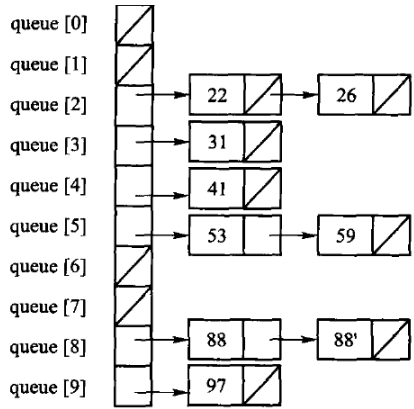
(d) 第二趟分配结果
