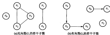
图 7.4 图 7.2 的若干子图: (a) 的两幅取自无向图 G_1 , (b) 的两幅取自有向图 G_2 。只保留一部分顶点和一部分边, 剩下的仍是原图的子图。
