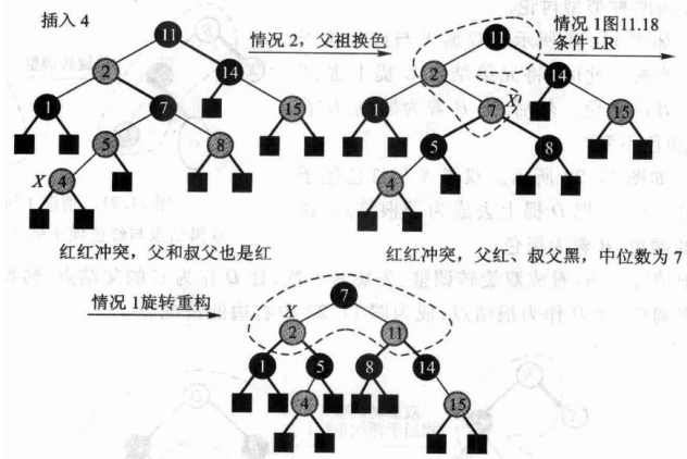
图 11.19 父与叔父都红：把父 A 和叔父 C 都改成黑、祖父 B 改成红。A 以下的冲突解决了，但 B 可能与它的父结点再冲突，于是把 B 当成新的 X 递归上去。最坏一路推到根，把根改回黑色即可——这是红黑树唯一会长高（阶加 1）的时刻。
