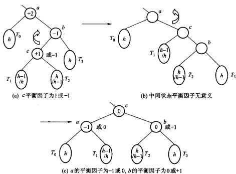
图 12.33 RL 型的双旋转, LR 型对称。中间那步的平衡因子没有意义 (图中的 (b)); 转完之后 a 的因子是 -1 或 0 、 b 的因子是 0 或 +1 , 取决于被提上来的那棵子树原来偏哪边。
