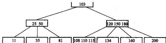
图 11.27 习题 9 的 4 阶 B 树
