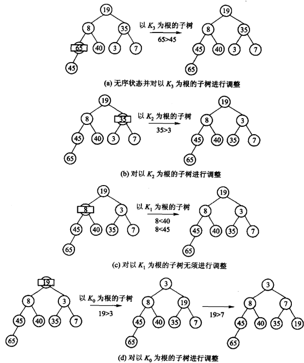
图 5.17 建堆过程示例（原书图 5.17 的筛选法）。倒着做的理由是：对某个结点下沉时，它的两棵子树必须已经是堆——从最后一个非叶结点往前扫，正好保证这一点。叶结点本身就是堆，所以后半一半结点一次都不用碰。
