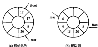
图 3.11 把数组看成环之后的样子：(a) 初始队列里有 12、17、8、20 四个元素；(b) 两次出队、三次入队之后，队列变成 8、20、15、9、6。入队增加 \text{rear} ，出队增加 \text{front} ，两者都在环上顺时针走。
