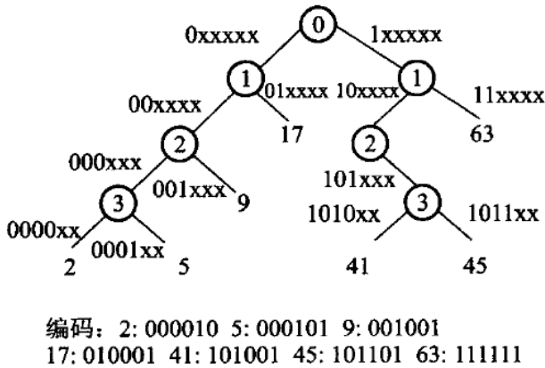
图 12.19 压缩的依据: x 表示该位取 0 取 1 都落在同一枝里, 也就是这一位不需要用来分支——把这样的层去掉就是 Patricia。
