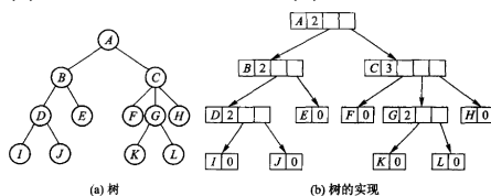
图 6.9 树的动态表示法：(a) 的每个结点在 (b) 里都是一块单独分配的空间，里面存着孩子数和一张长度可变的孩子指针表。
