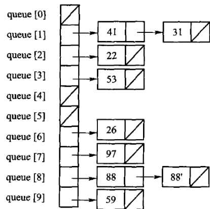
(b) 第一趟分配结果
