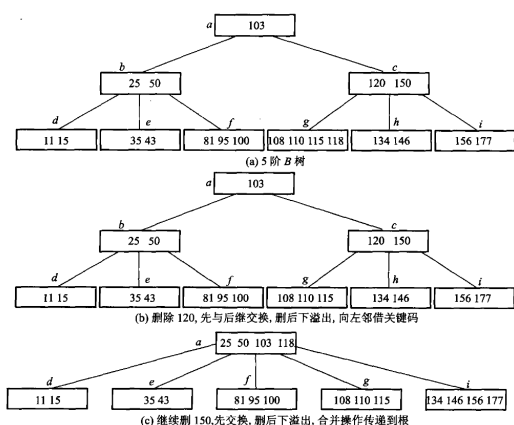
图 11.8 在一棵 (a) 5 阶 B 树上连续删除: (b) 删 120——先与中序后继交换再删, 删后下溢, 向左邻借一个关键字; (c) 接着删 150——同样先交换, 删后下溢而两侧都借不到, 只能合并, 合并又让父结点下溢, 一路传到根。
