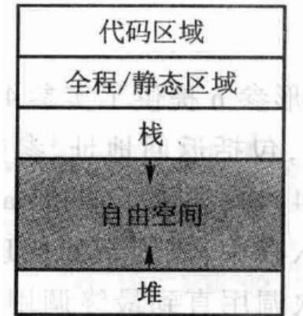
图 3.6 运行时存储器的组织形式：栈区放具有后进先出特征的数据（函数调用），堆区放不符合 LIFO 的动态分配（例如 new 出来的对象）。
