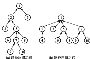
图 6.13 查找根结点时把沿途父指针直接改到根：(a) 是压缩之前的树，(b) 是对结点 7 调用一次 find 之后的样子——路径 7 \rightarrow 5 \rightarrow 2 上的结点都被直接改挂到根 1 下，而 9、10 仍留在 7 下面。
