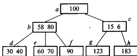
图 11.28 习题 10 的 3 阶 B 树
