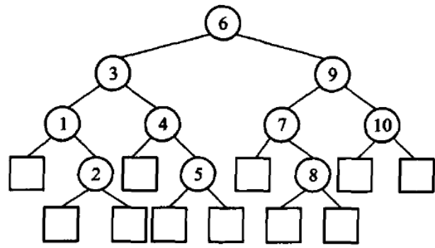
图 5.3 扩充二叉树：方框是补出来的外部叶，圆圈是原有的内部结点。补完之后每个内部结点都恰好有两个孩子，所以扩充二叉树一定是满二叉树——5.6 节算带权外部路径长度时用的就是这张图的形状。设内部路径长度 I 为根到所有内部结点的边数之和，外部路径长度 E 为根到所有外部叶的边数之和，则
