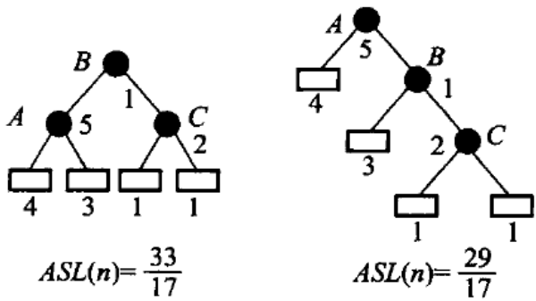
图 12.26 结点权不等时，最佳的形状未必最平衡：权大的关键字要往根靠，哪怕整棵树因此歪一些。这正是需要动态规划、而不是简单「取中位数当根」的原因。
