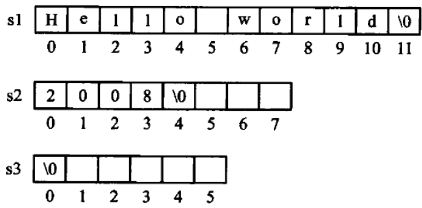
图 4.1 C 风格字符串的变量说明示意。'\0' 是 ASCII 里 8 位全 0 的 NULL 符，只作结束标记用，不算内容；说明变量时可以用字符串常量给初值，也可以不给——图中的 s3 没给初值，存的就是空串。
