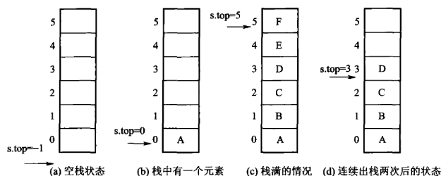
图 3.3 顺序栈的存储结构：(a) 空栈， \text{s.top} = -1 ；(b) 栈中有一个元素， \text{s.top} = 0 ；(c) 栈满， \text{s.top} = \text{mSize} - 1 ；(d) 在 (c) 上连续出栈两次之后的状态。
