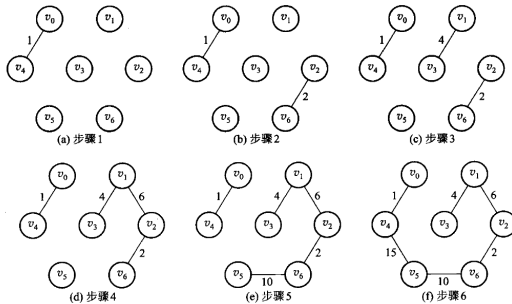
图 7.25 Kruskal 算法在同一张图 7.23 上的步骤（同样跨两页，(a)(b)(c) 与 (d)(e)(f) 各一张）。中间过程是一片森林，直到最后才连成一棵树；判断「这条边会不会成环」就是判断两个端点是不是已经在同一棵树里——这正是第 6 章并查集的用处。两个算法走的路不同，得到的总权相同。
