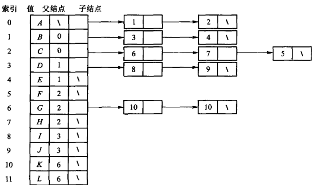
图 6.6 每个结点单独保存孩子表的表示法。
