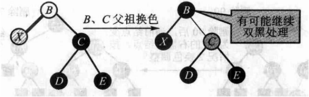
图 11.23 只换色：兄弟 C 着红、父 B 着黑。B 原来是红的就此结束；原来是黑的，就把 B 当成新的双黑继续往上调整。
