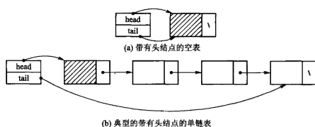
图 2.6 引入头结点的单链表：(a) 带头结点的空表，(b) 一个典型的带头结点的单链表。带阴影的那个结点就是头结点，它的数据域不算表中元素，只是为了让空表和表头不再是特例。
