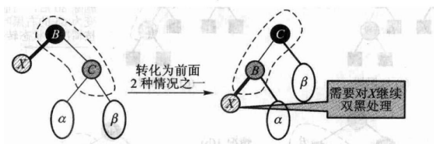
图 11.24 此时父结点必为黑、兄弟的两个孩子必为黑。旋转一次之后 X 仍是双黑，但已经化归成前两种情况，继续处理即可。
