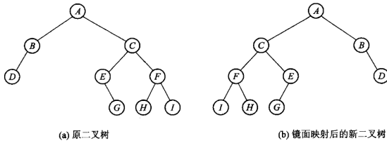
图 5.22 习题 7 的图例：(a) 原二叉树，(b) 镜面映射后的新二叉树
